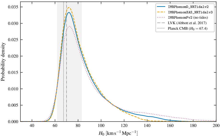
GW170817 H_0 posterior — waveform comparison
