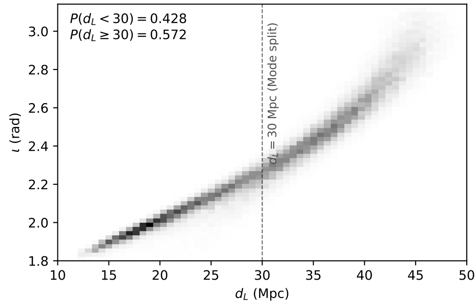
IMR/NRTidalv2 (refModeB)
