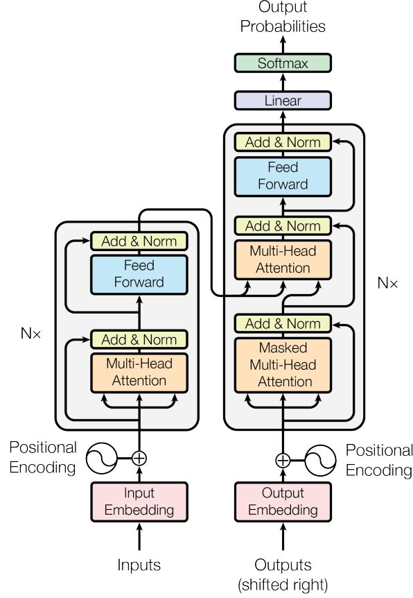
Figure 1: The Transformer - model architecture. 变压器 - 模型架构。
