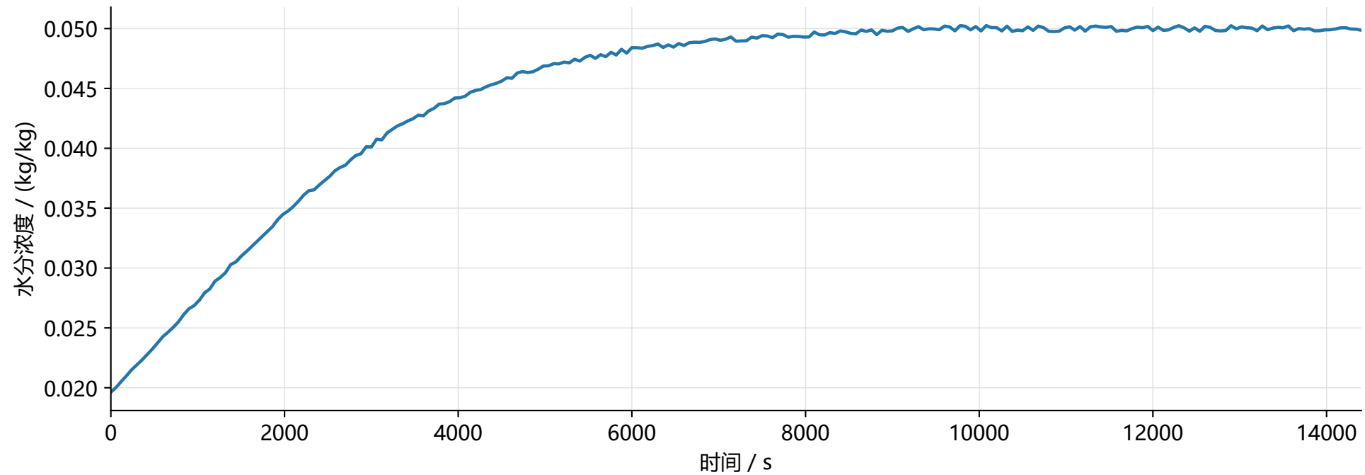
附件一：烘房水分浓度随时间的变化
