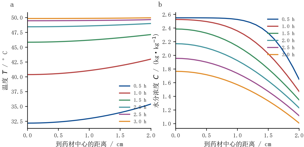
图3 3 小时内温度与水分浓度沿径向的分布
