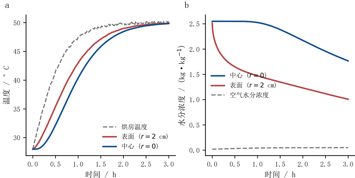
图4 中心与表面温度、水分浓度随时间的演化
