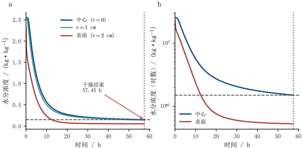
图7 中心与表面水分浓度随时间的变化
