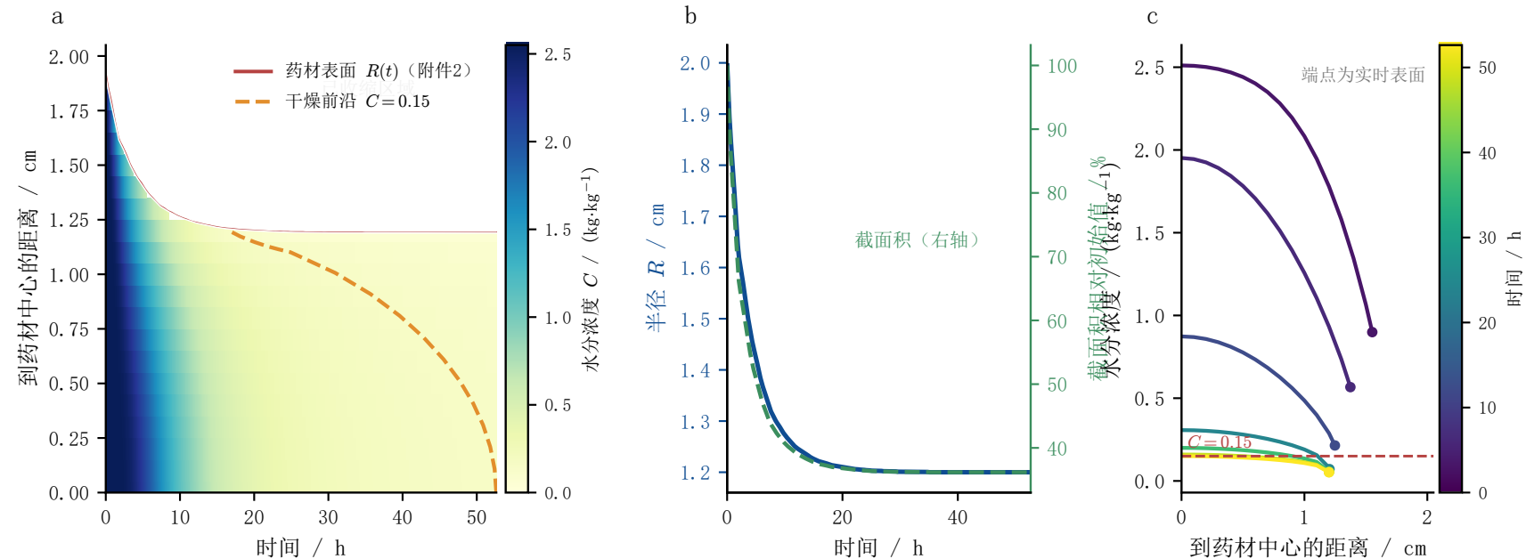
图E 收缩域内水分浓度的时空演化（问题4）
