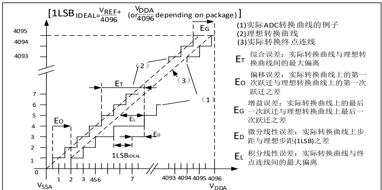
图 23. ADC 精度特性
