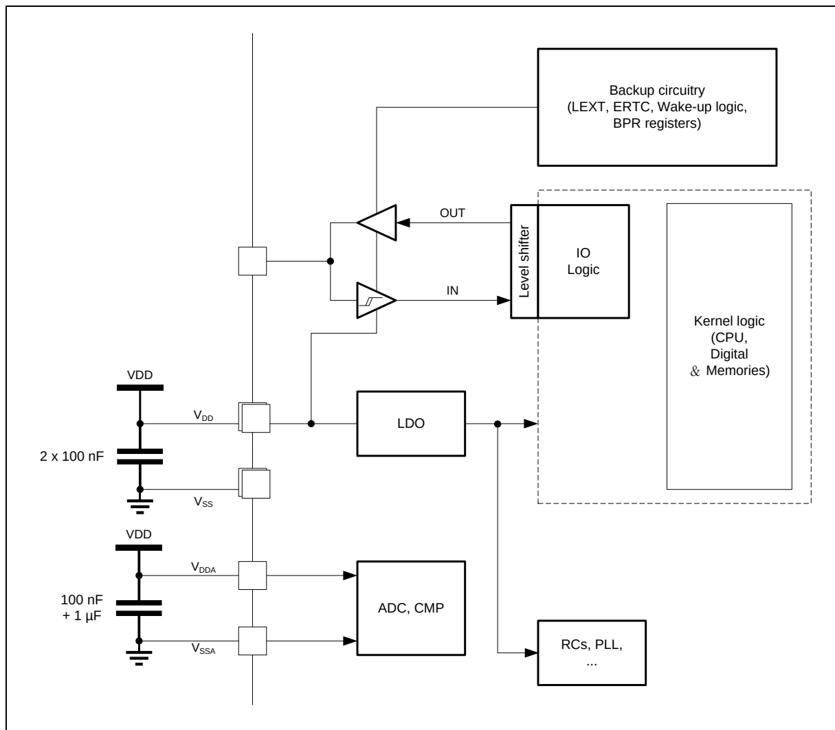
图 7. 供电方案
