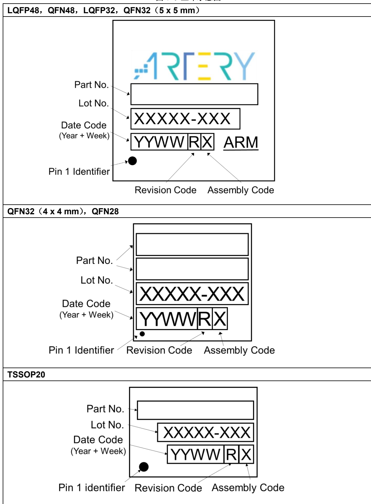
图 34. 丝印示意图
