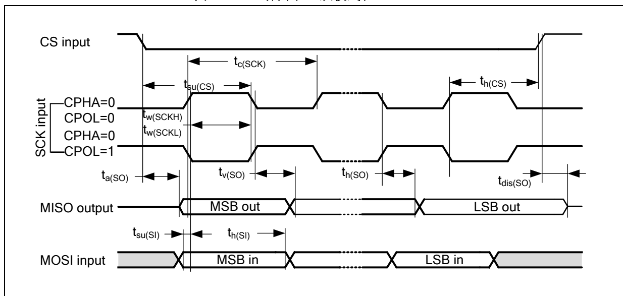
图 18. SPI 时序图 - 从模式和 CPHA = 0
