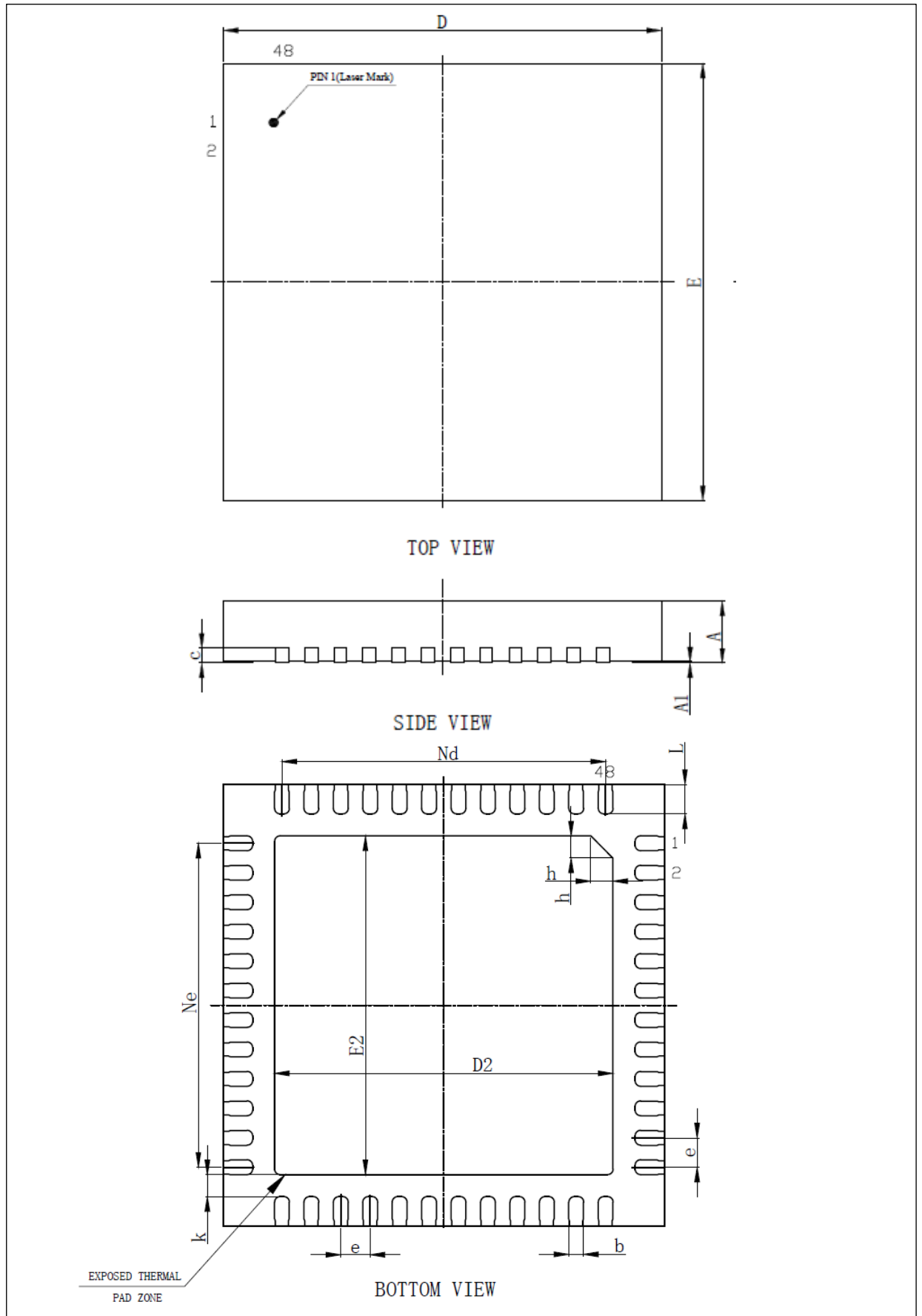
图 28. QFN48 – 6 x 6 mm 48 引脚正方扁平无引线封装图
