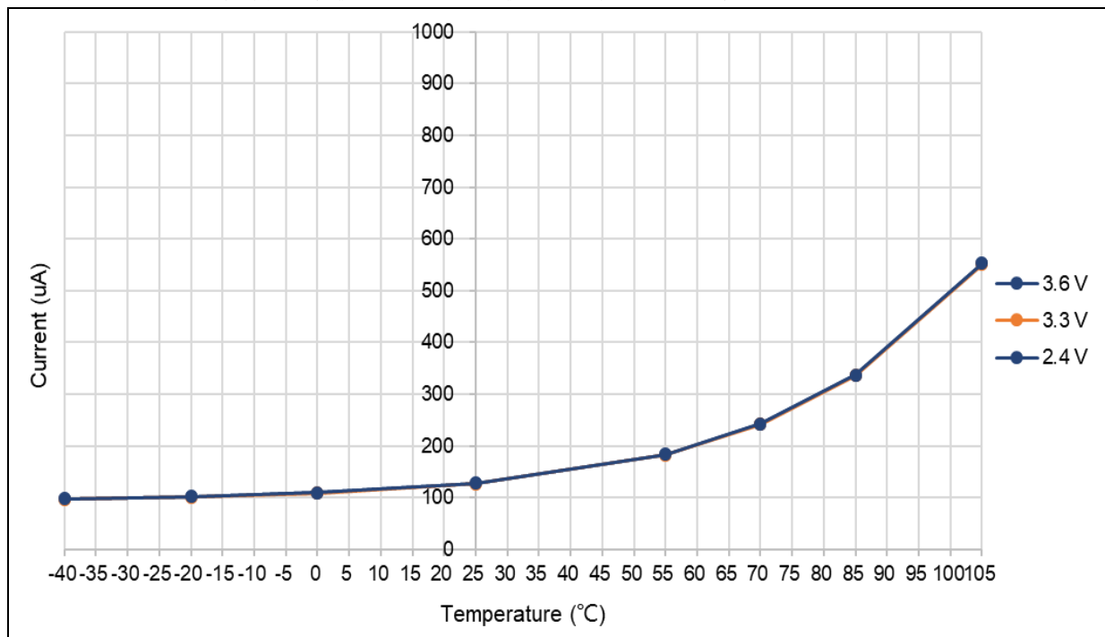
图 11. 待机模式下的典型电流消耗在不同的 V_{DD} 时与温度的对比
