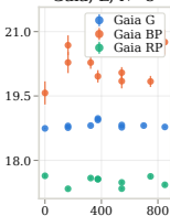
Gaia, E, N=8
