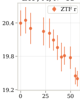
ZTF, M, N=19
