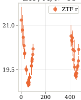
ZTF, M, N=20
