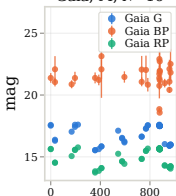
Gaia, M, N=16
