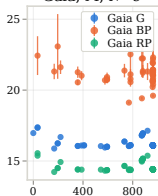
Gaia, M, N=14
