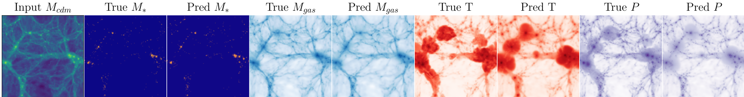
IllustrisTNG
