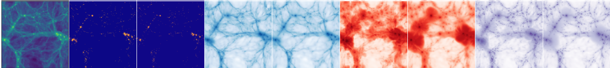
Magneticum
