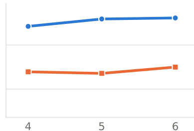
MLP
