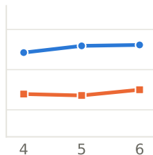
MLP
