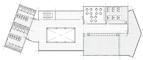
<그림 6> 3층 & 4층 평면도
