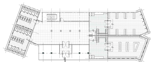
<그림 4> 1층 평면도
