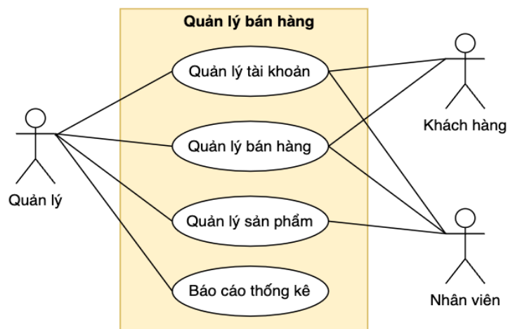
Hình 4: Biểu đồ Usecase Tổng quan hệ thống.
