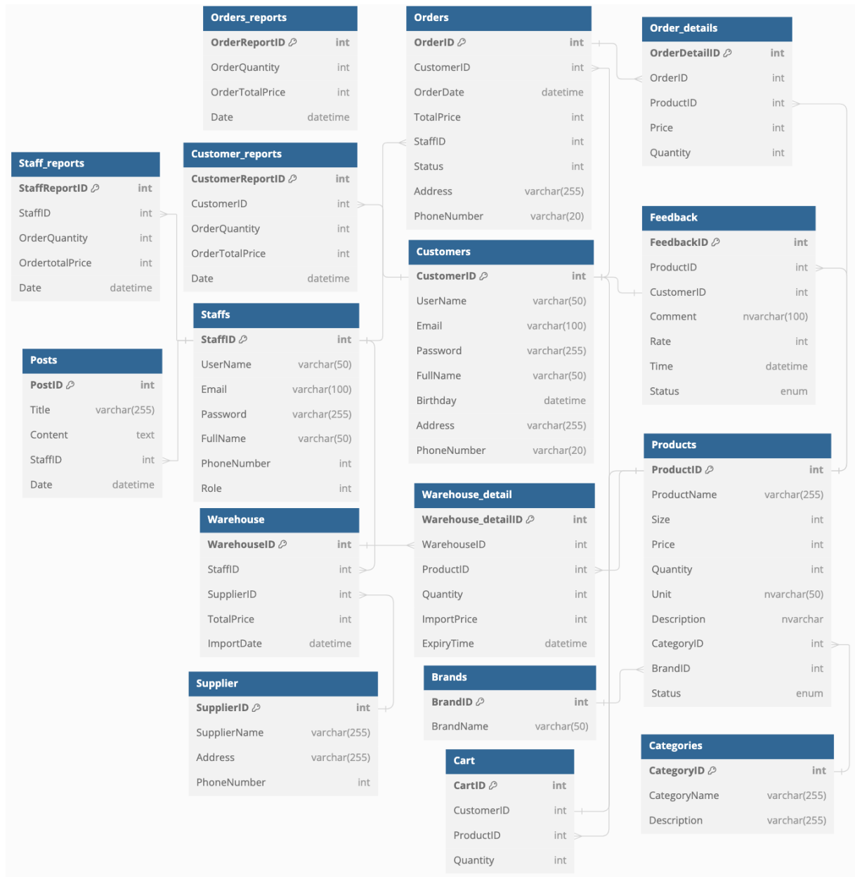
Hình 24: Biểu đồ ERD.
