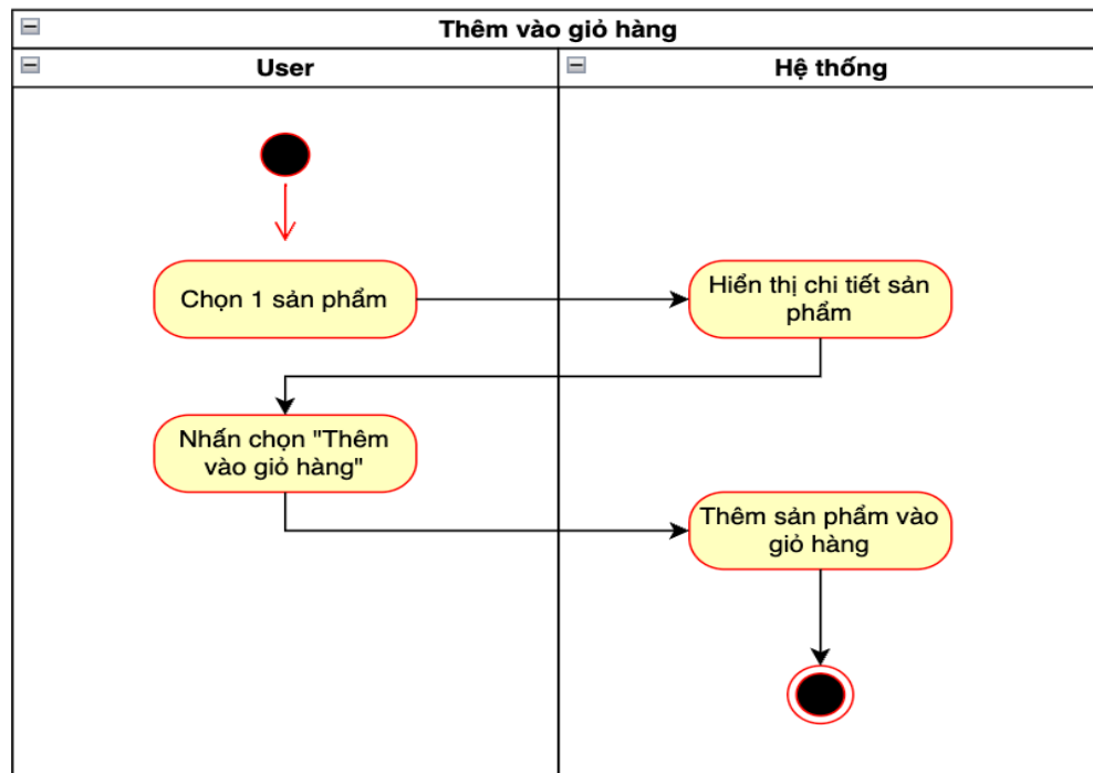
Hình 13: Biểu đồ Hoạt động Use Case “Thêm vào giỏ hàng”.
