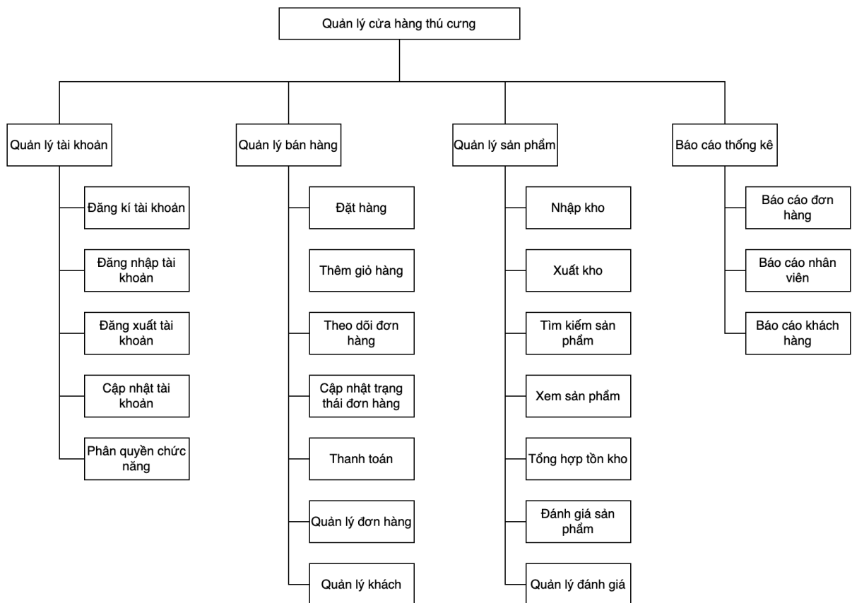
Hình 3: Sơ đồ phân cấp chức năng.
