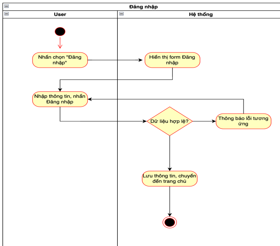
Hình 10: Biểu đồ Hoạt động Use Case “Đăng nhập”.
