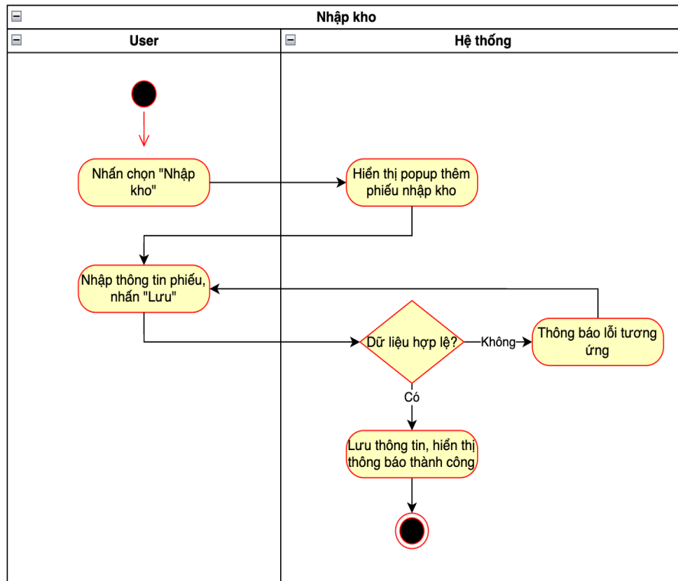
Hình 17: Biểu đồ Hoạt động Use Case “Nhập kho”.
