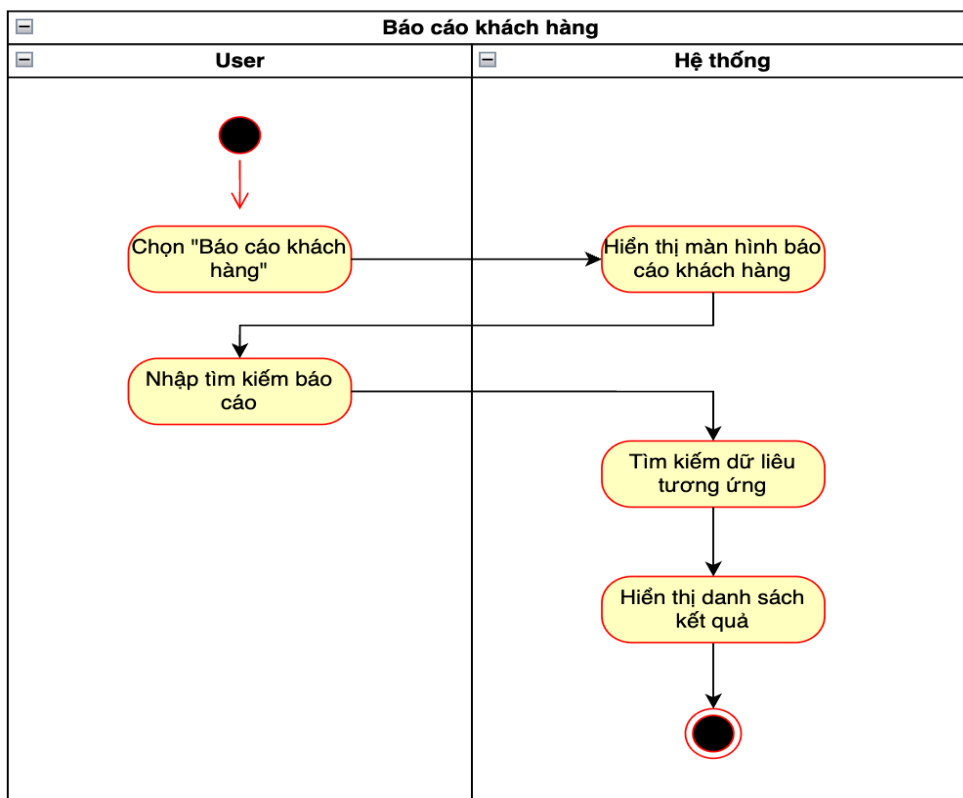
Hình 22: Biểu đồ Hoạt động Use Case “Báo cáo khách hàng”.
