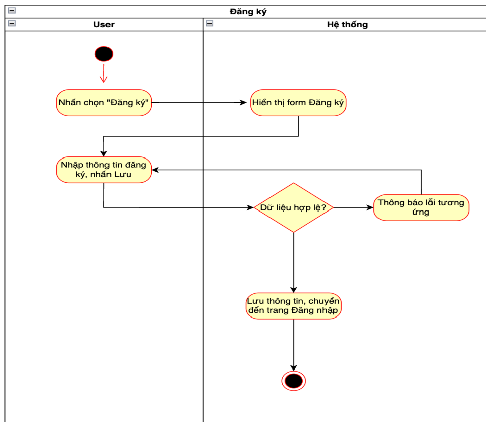
Hình 9: Biểu đồ Hoạt động Use Case “Đăng ký”.
