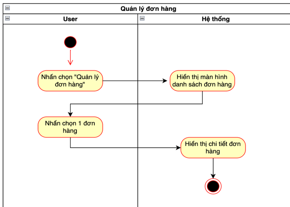
Hình 16: Biểu đồ Hoạt động Use Case “Quản lý đơn hàng”.
