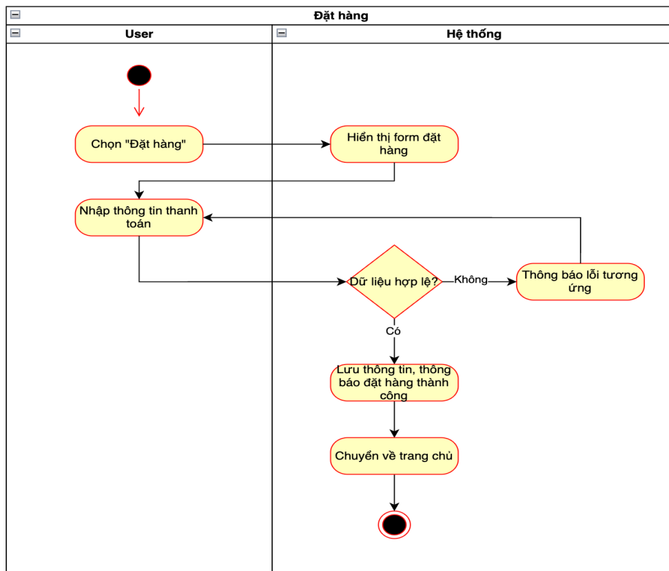
Hình 12: Biểu đồ Hoạt động Use Case “Đặt hàng”.
