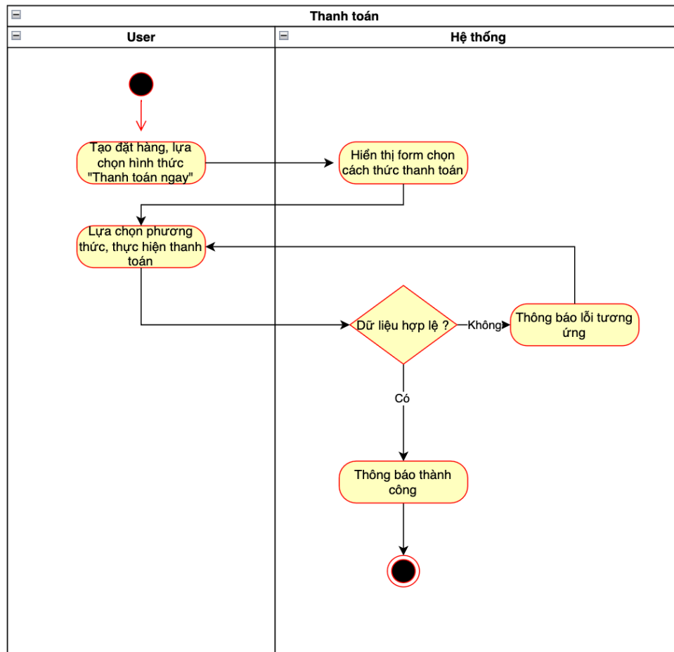
Hình 15: Biểu đồ Hoạt động Use Case “Thanh toán”.
