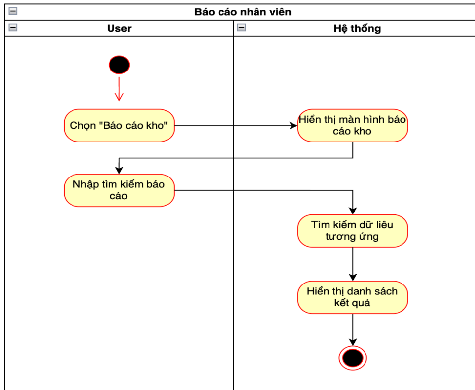
Hình 21: Biểu đồ Hoạt động Use Case “Báo cáo nhân viên”.
