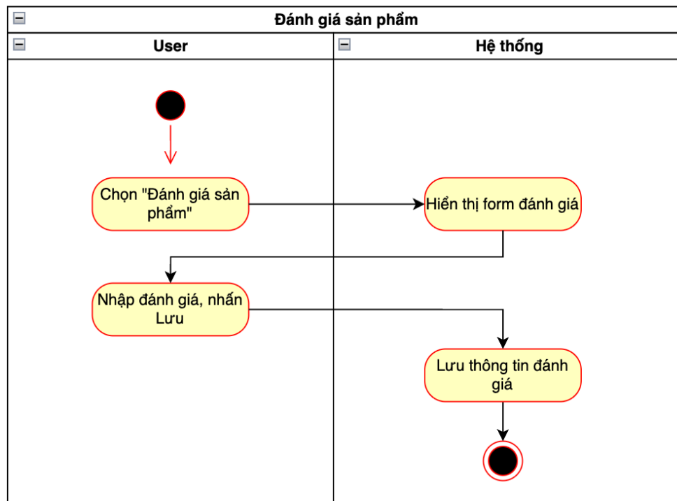
Hình 18: Biểu đồ Hoạt động Use Case “Đánh giá sản phẩm”.
