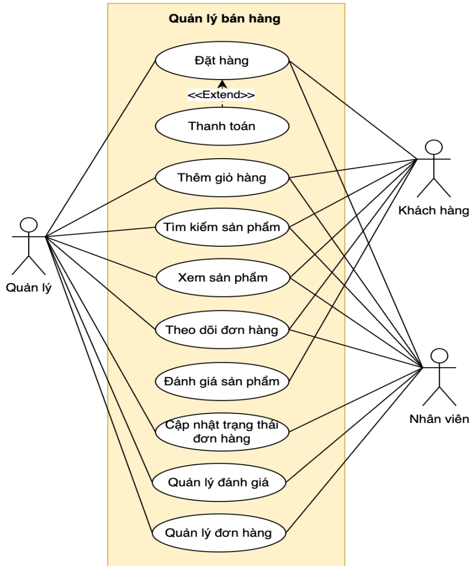
Hình 6: Biểu đồ Usecase Quản lý bán hàng.
