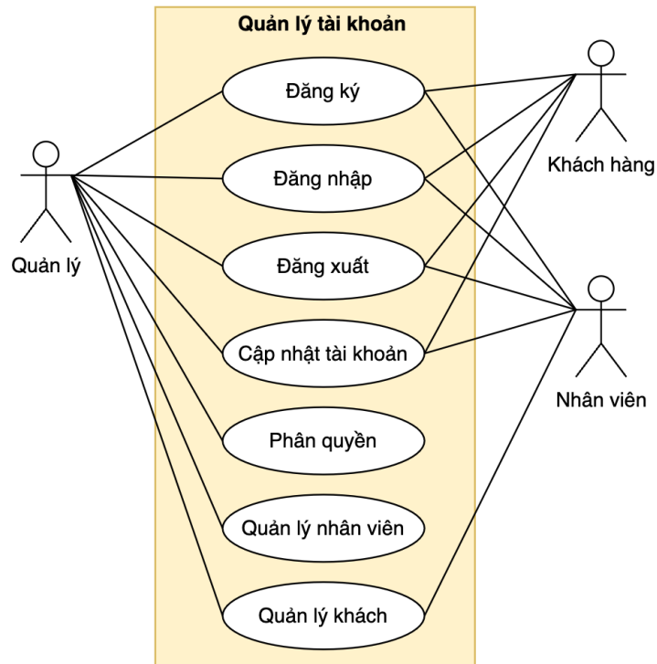
Hình 5: Biểu đồ Usecase Quản lý tài khoản.
