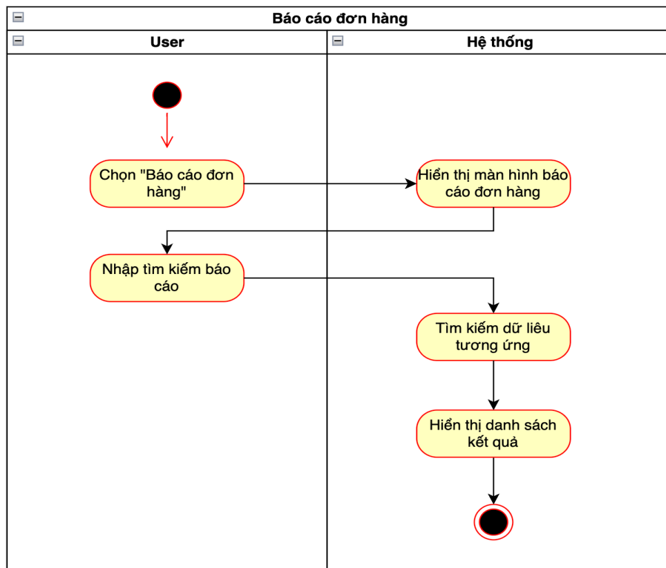
Hình 20: Biểu đồ Hoạt động Use Case “Báo cáo đơn hàng”.
