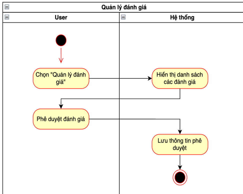
Hình 19: Biểu đồ Hoạt động Use Case “Quản lý đánh giá”.
