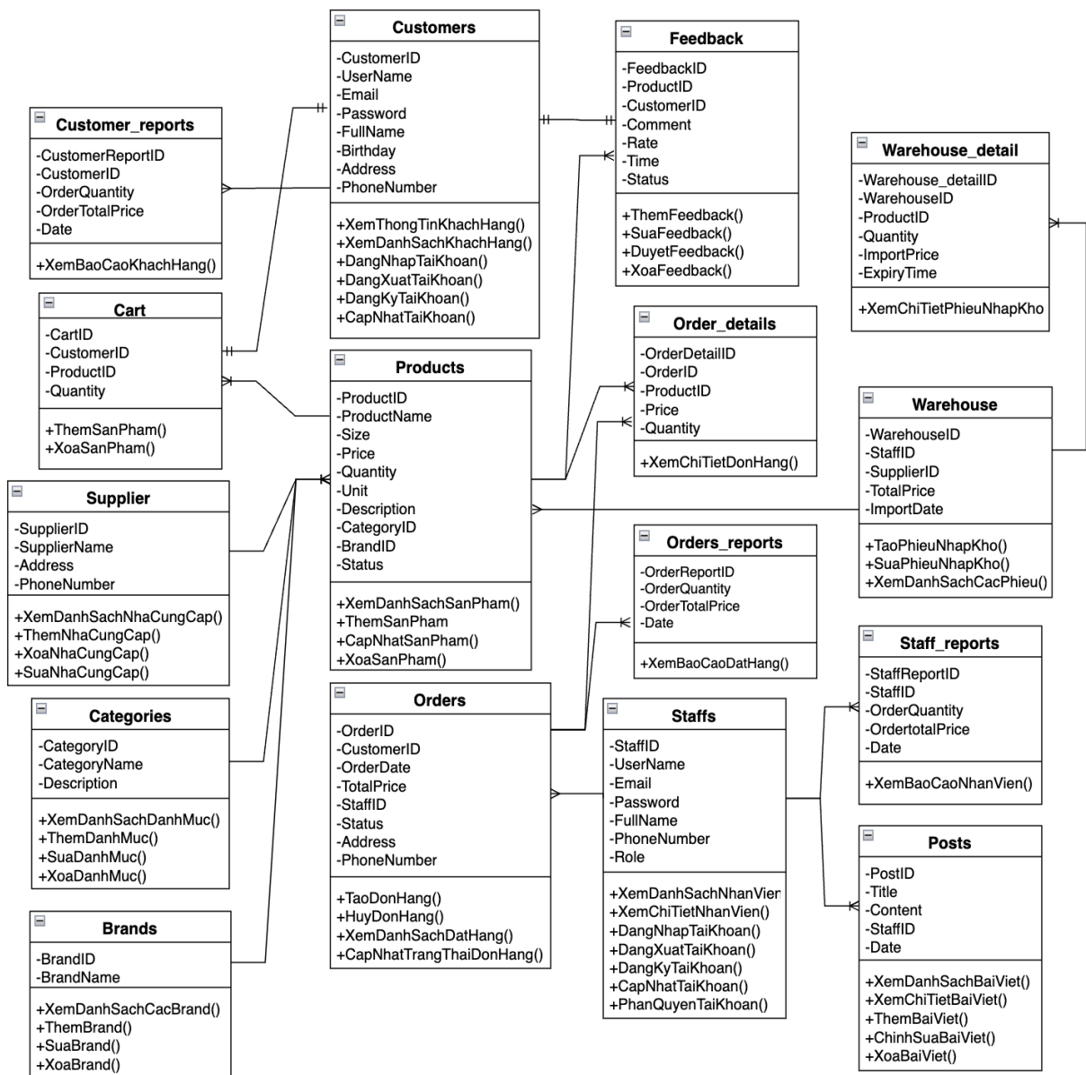
Hình 23: Biểu đồ lớp.
