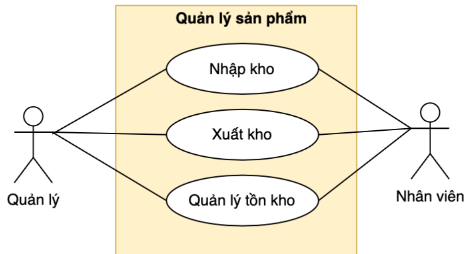
Hình 7: Biểu đồ Usecase Quản lý sản phẩm.
