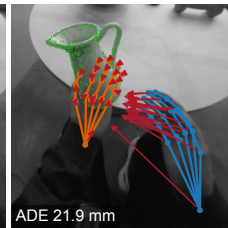
factored (FIF)
