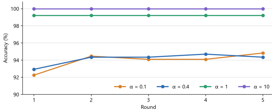
Hình 9. Accuracy của mô hình toàn cục qua các round với các mức \alpha khác nhau (seed = 7)
