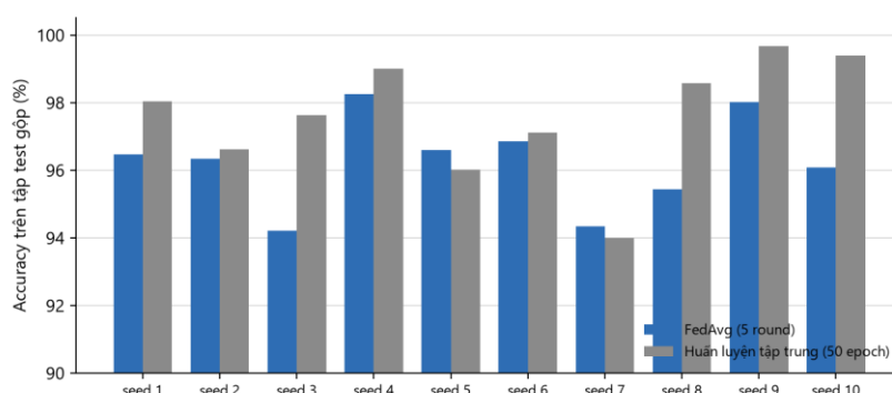
Hình 8. Accuracy của FedAvg và huấn luyện tập trung trên 10 seed dữ liệu
