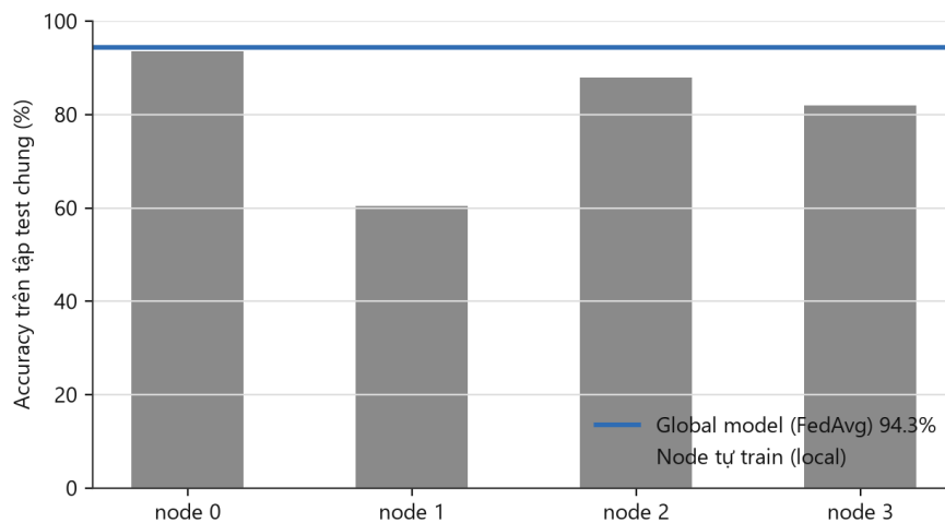
Hình 7. Mô hình toàn cục (FedAvg) so với từng nút tự huấn luyện, trên tập kiểm tra chung
