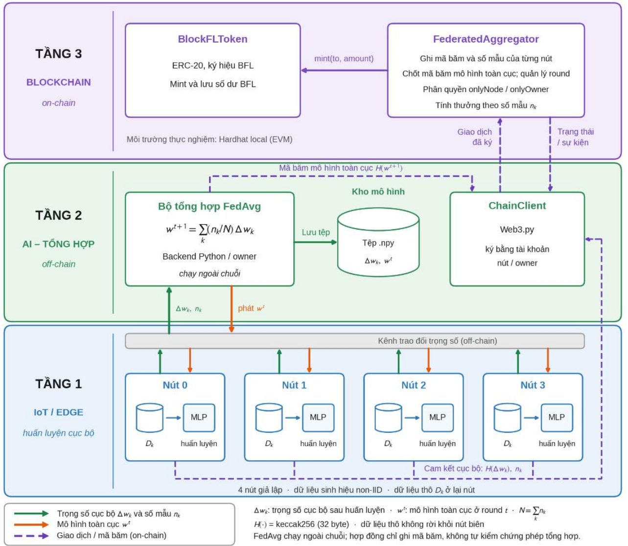
Hình 1. Kiến trúc 3 tầng CPS: IoT \rightarrow AI (Federated Learning) \rightarrow Blockchain
