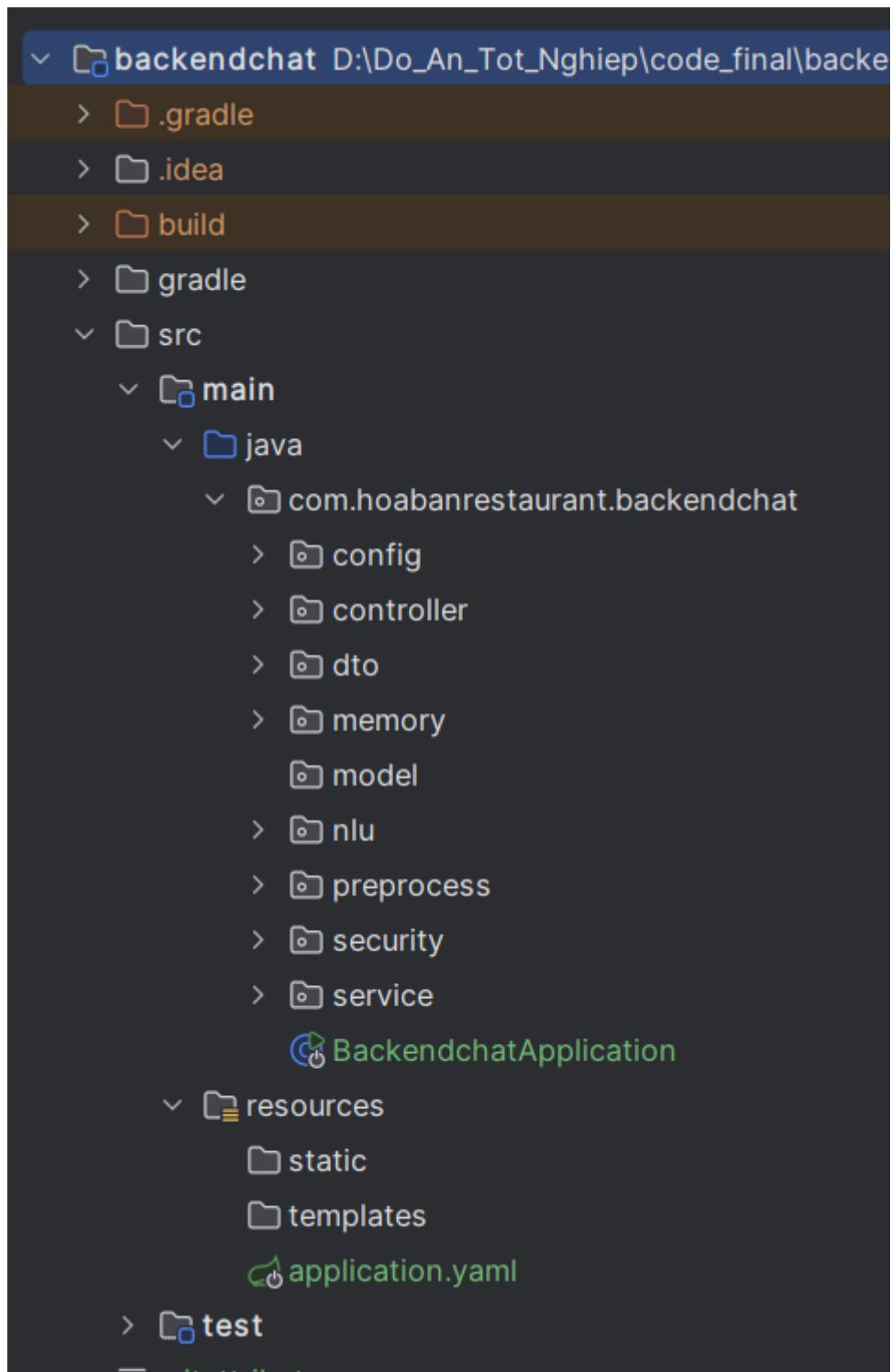
Hình 4-2: Cấu trúc thư mục backend chatbot
