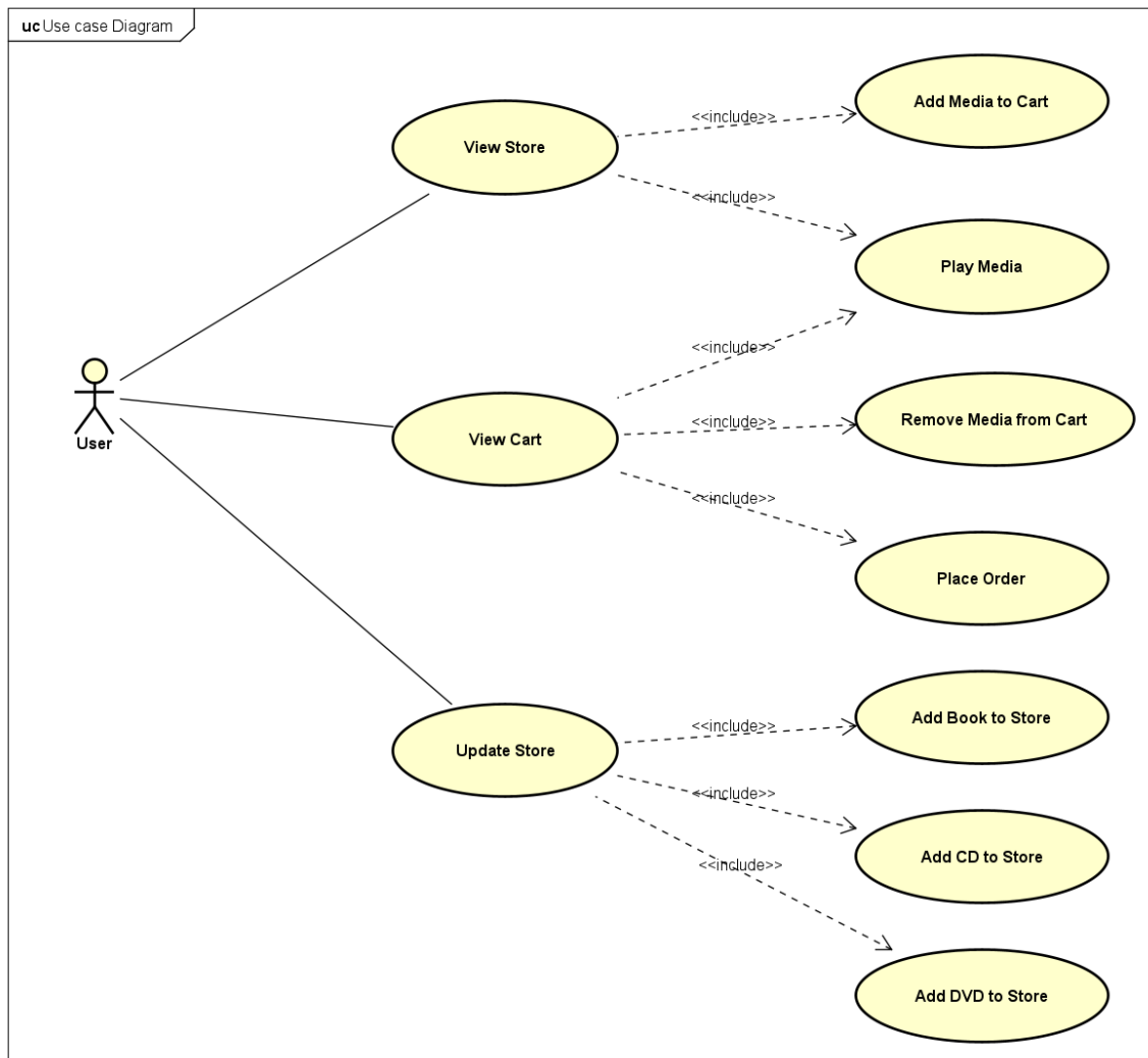
Hình 4: Use case diagram của AIMS trong Lab 05
