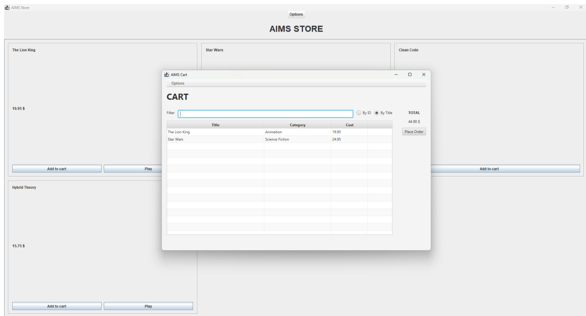
Hình 3: Màn hình CartScreen
