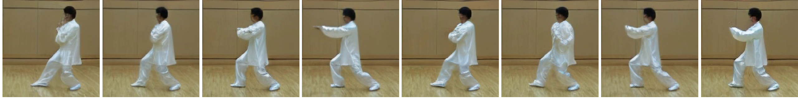
FrameDiT-G
