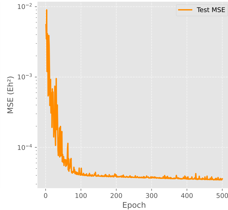
MSE
