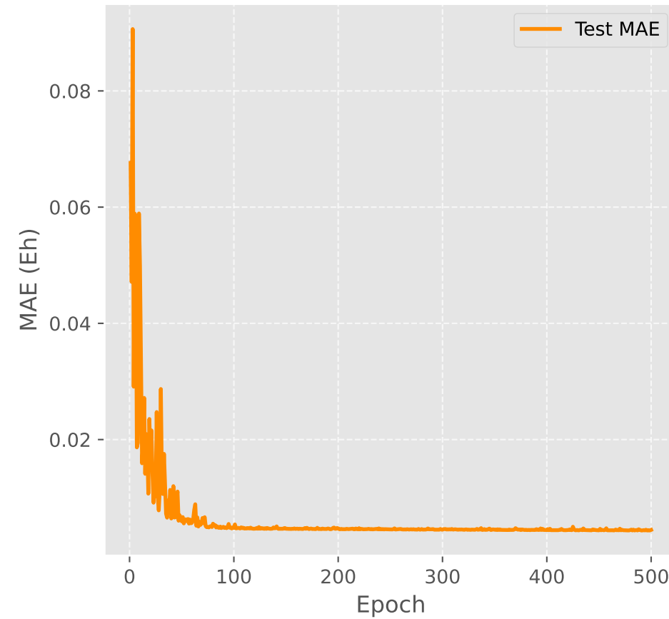
MAE
