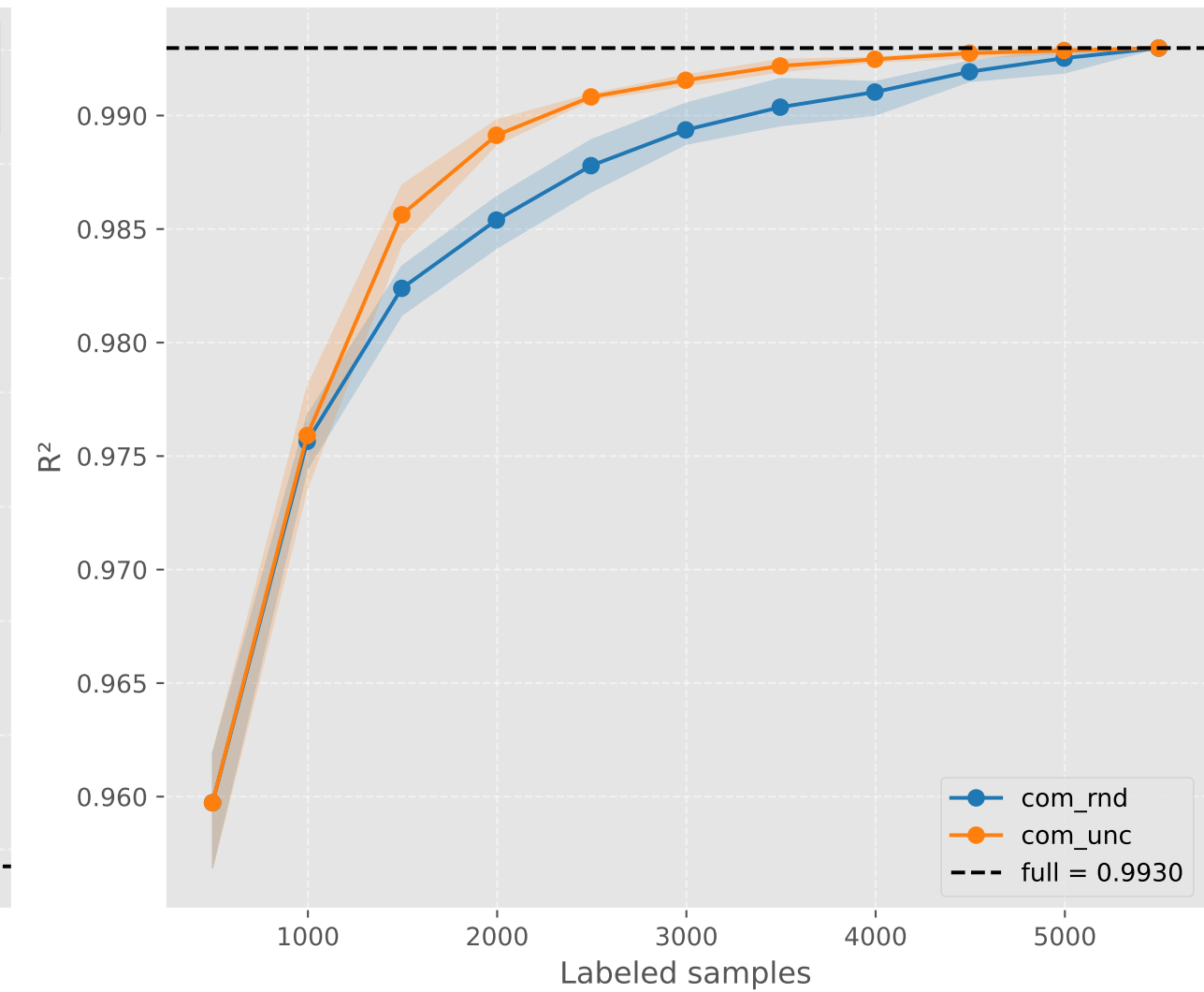
R^2
