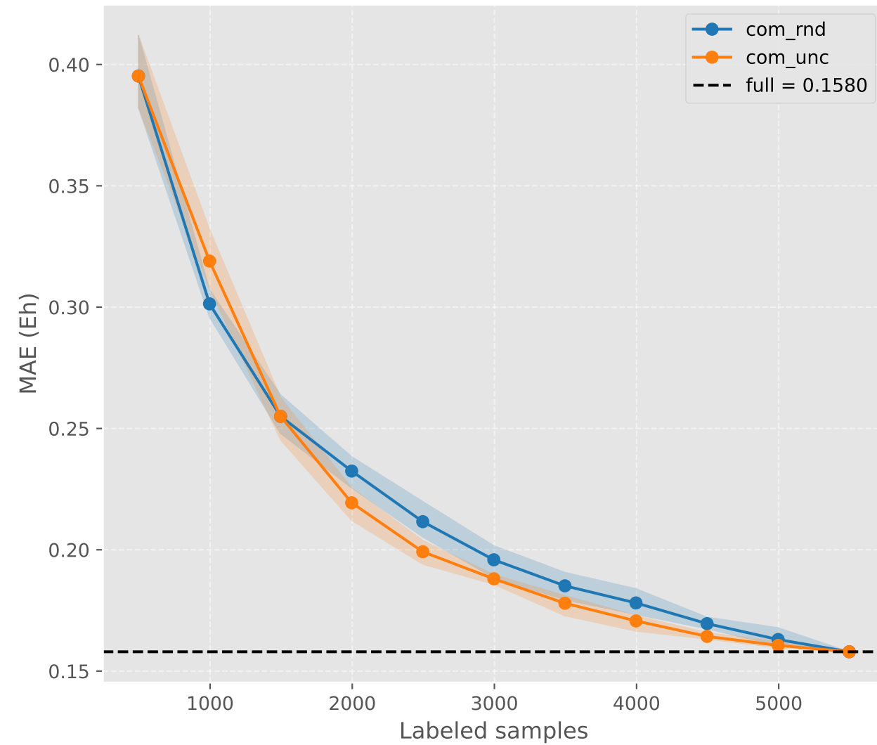
MAE (Eh)
