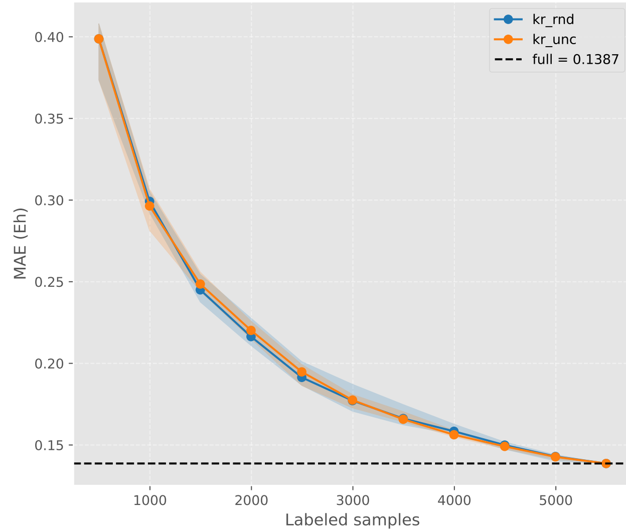
MAE (Eh)
