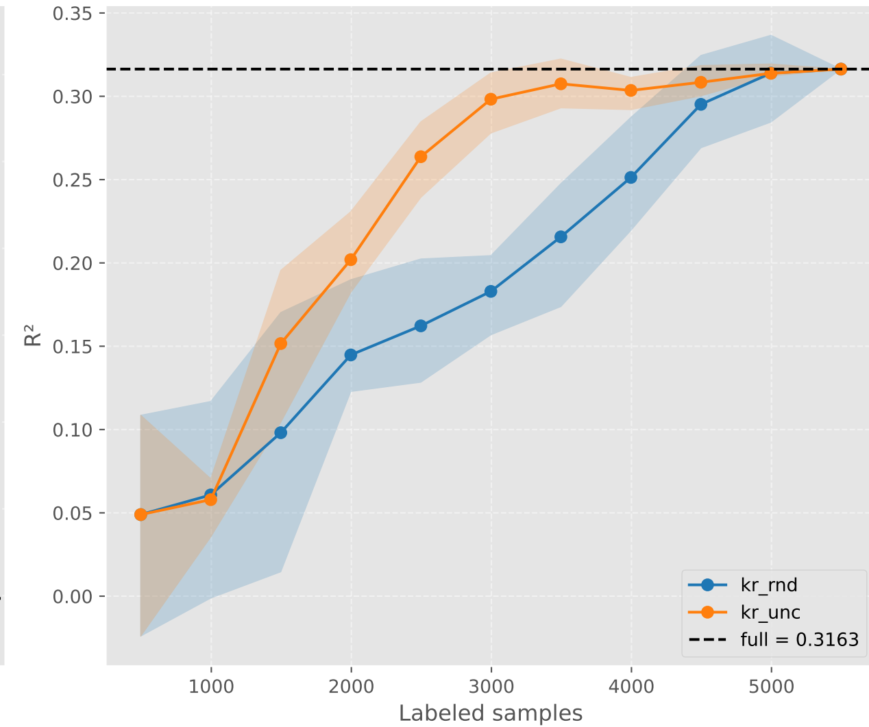
R^2
