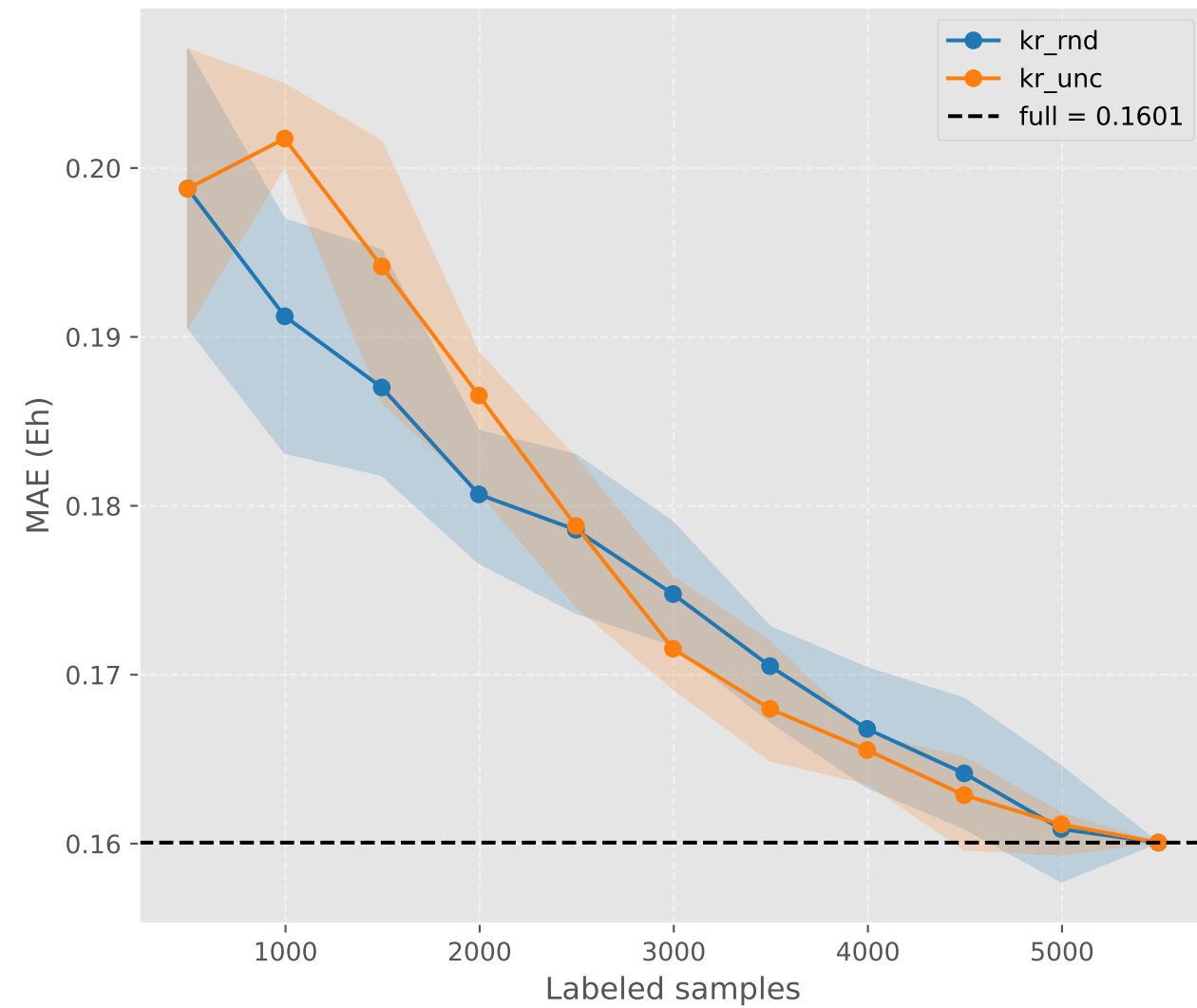
MAE (Eh)
