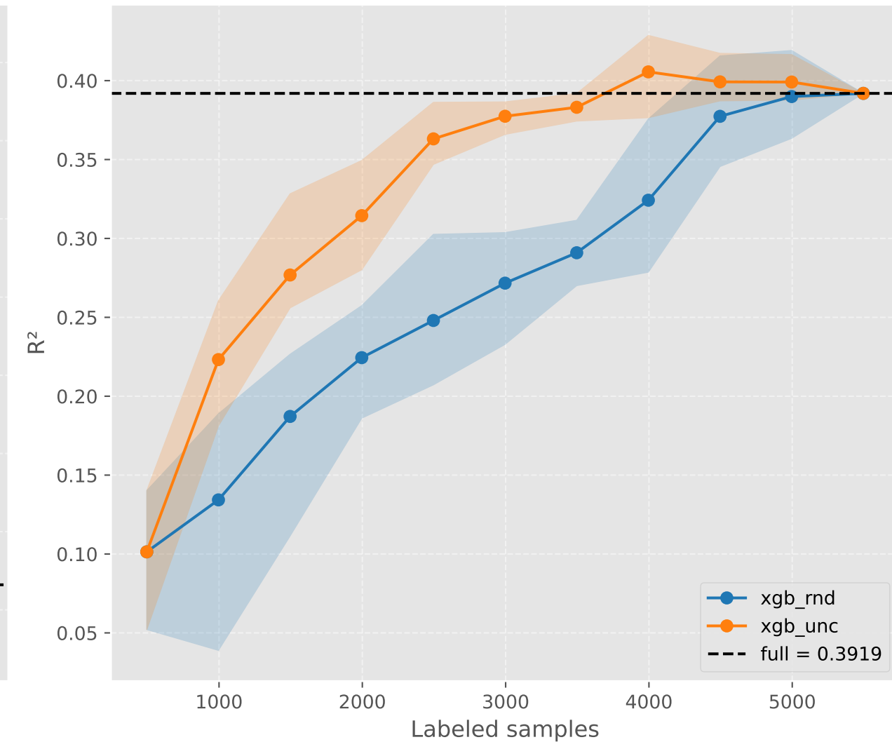
R^2
