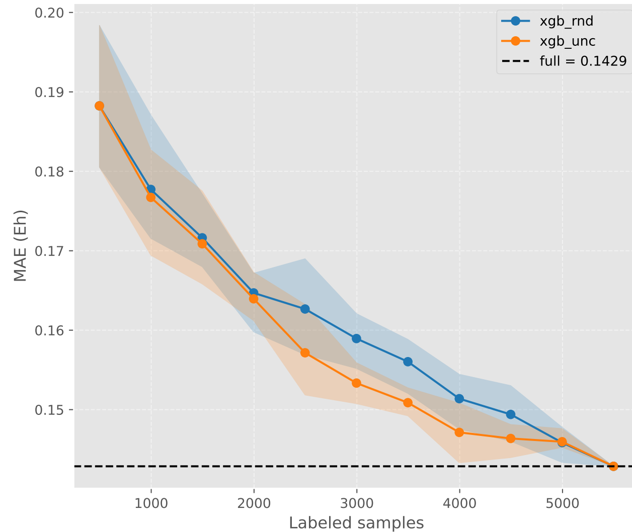
MAE (Eh)
