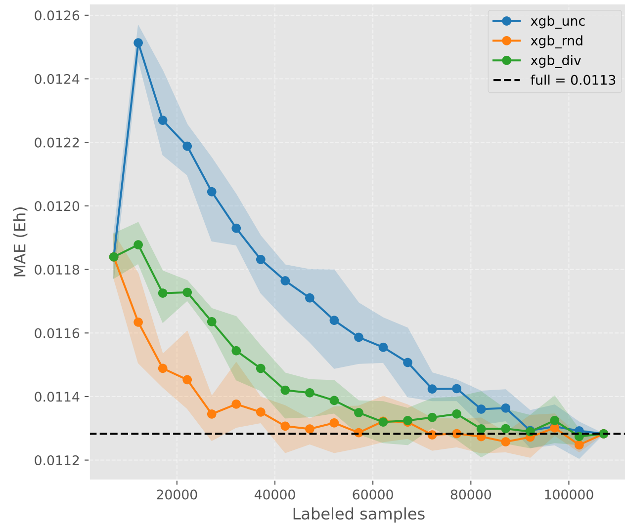
MAE (Eh)
