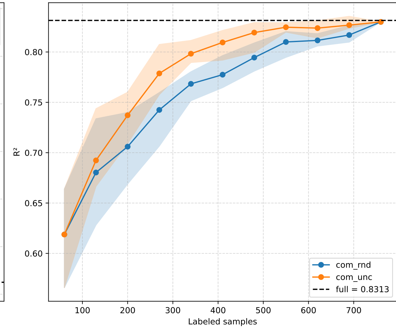
R^2
