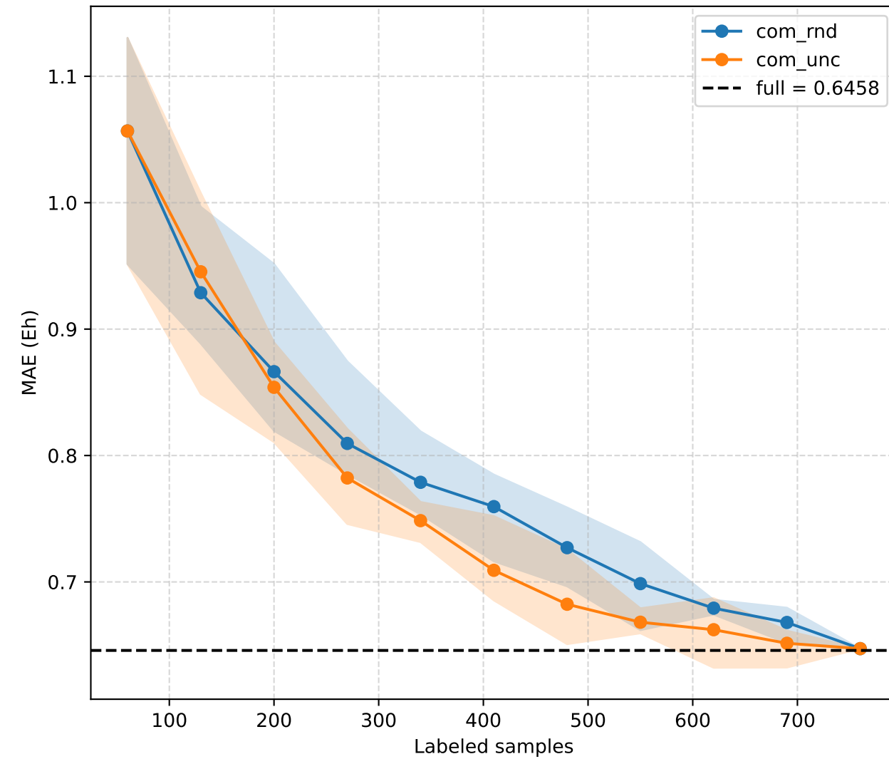
MAE (Eh)
