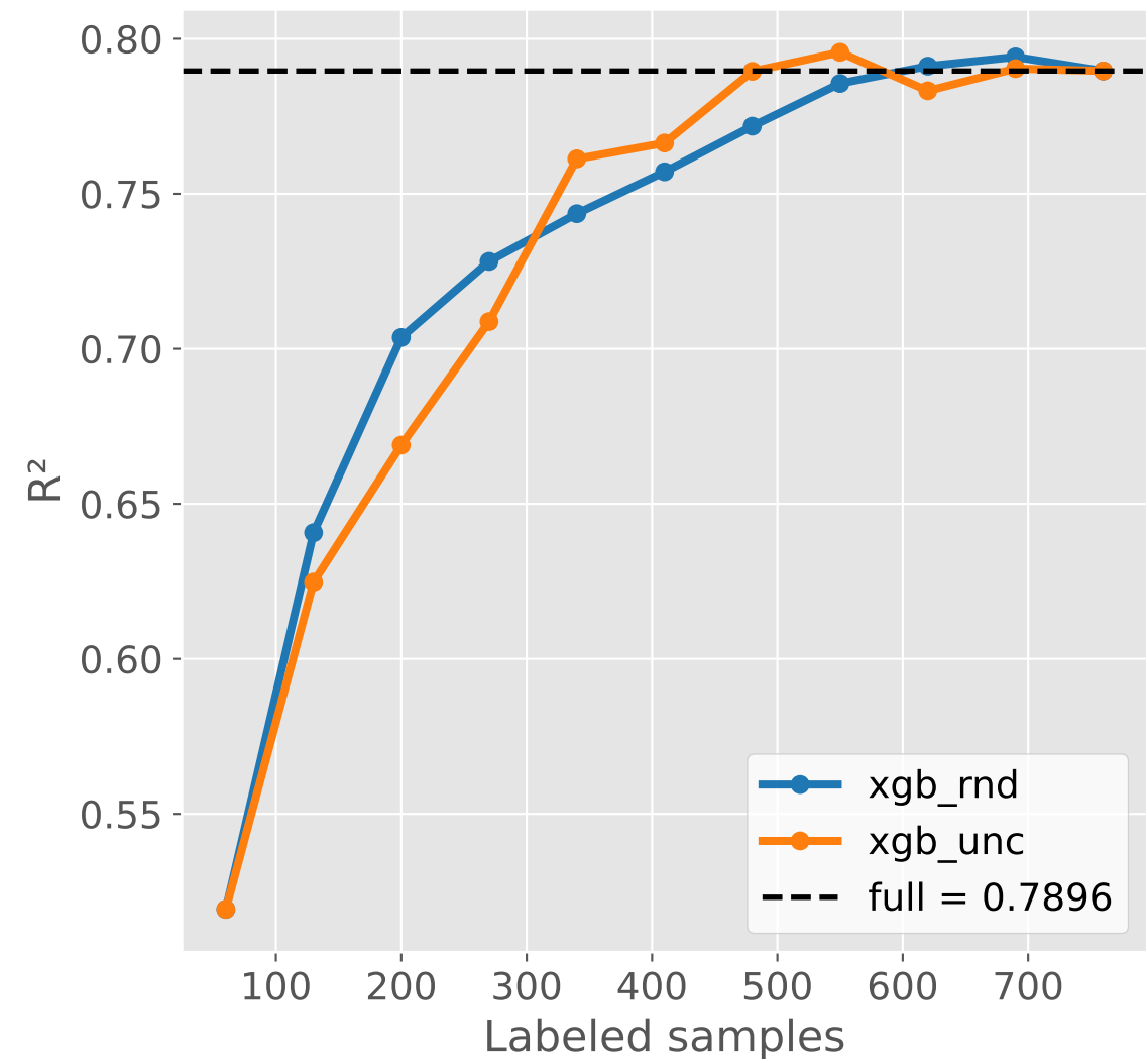
R^2
