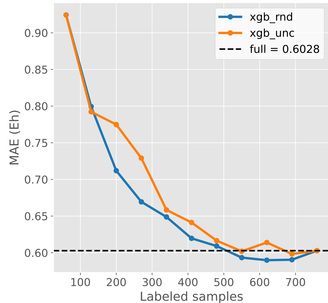
MAE (Eh)
