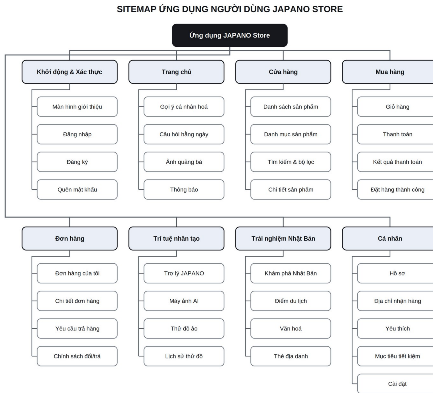
Hình 4.9: Sitemap ứng dụng người dùng JAPANO Store
