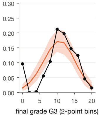
(b) Model 2: posterior predictive
