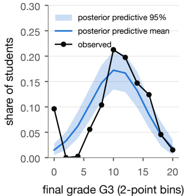
(a) Model 1: posterior predictive
