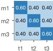
A: true p
