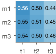
B: true p
