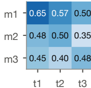
C: true p
