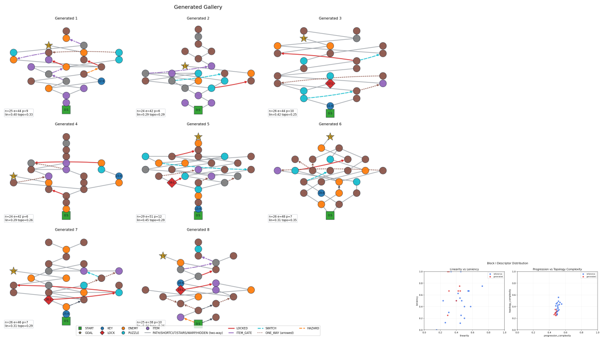
Hình 4.7: Kết quả sinh đồ thị Block I từ pipeline thật (seed 42, 8 đồ thị sinh): trái là gallery đồ thị nhiệm vụ được sinh, phải là phân bố descriptor của tập sinh so với tập tham chiếu. Hình được xuất trực tiếp từ pipeline đánh giá, không dùng topology vẽ tay.
