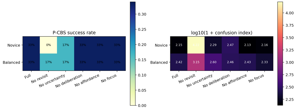
Hình 4.6: Tổng hợp ablation P-CBS trên hai hồ sơ persona đã hoàn tất đầy đủ. Biểu đồ trái cho thấy tỉ lệ thành công; biểu đồ phải biểu diễn chỉ số rối trí sau biến đổi \log_{10}(1 + x) để các biến thể có thể được đọc trên cùng một thang màu.
