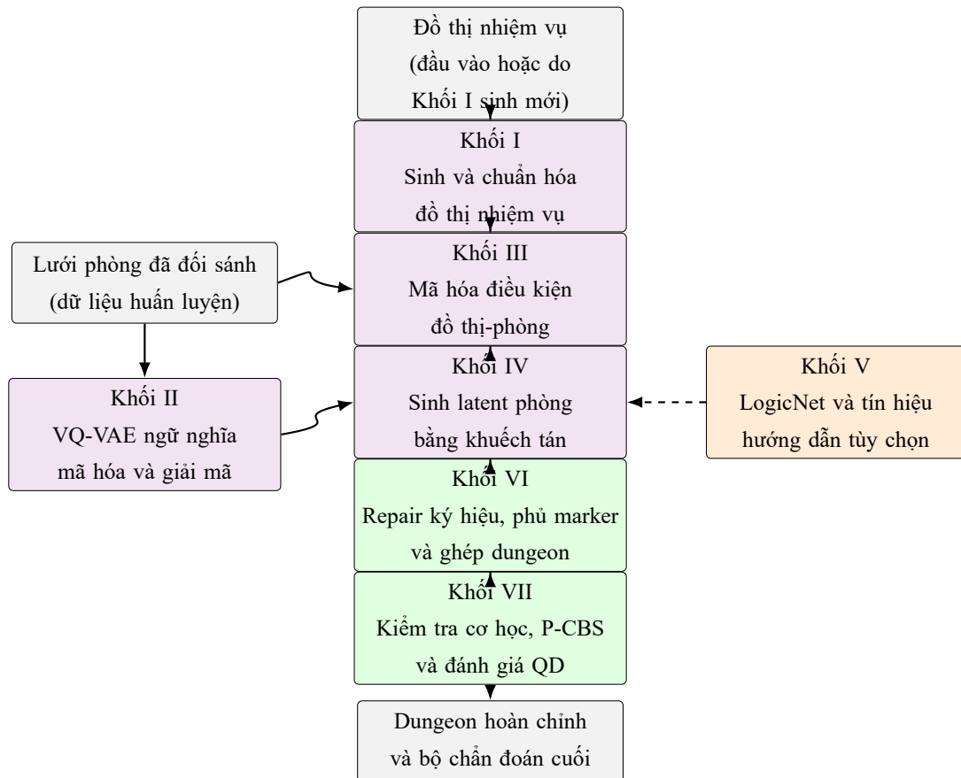
Hình 3.2: Kiến trúc bảy khối của quy trình sinh lại nơ-ron – ký hiệu theo hướng lấy đồ thị nhiệm vụ làm trung tâm. Trục dọc ở giữa là đường chạy lõi từ đồ thị nhiệm vụ đến dungeon hoàn chỉnh; nhánh trái là lớp học biểu diễn và nhánh phải là tín hiệu logic tùy chọn.
