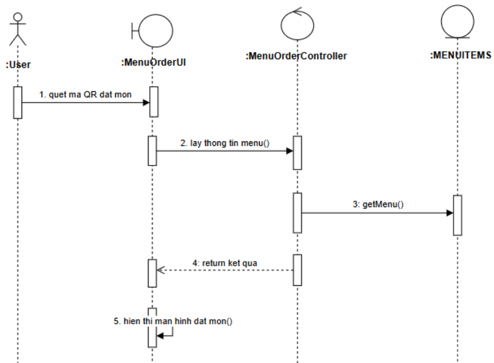
Hình 2.10: Biểu đồ trình tự use case Quét QR đặt món
