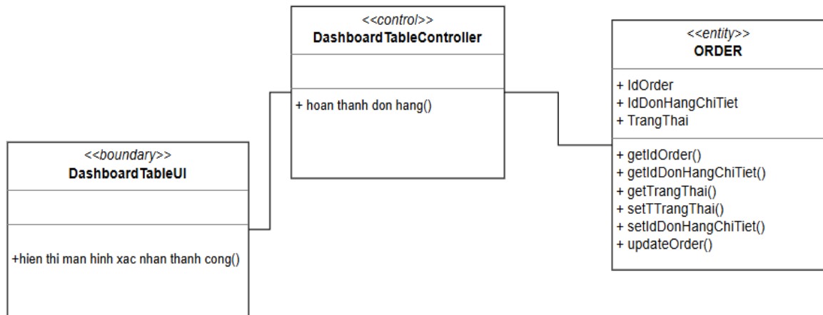
Hình 2.33: Biểu đồ VOPC use case Xác nhận đơn đặt món
