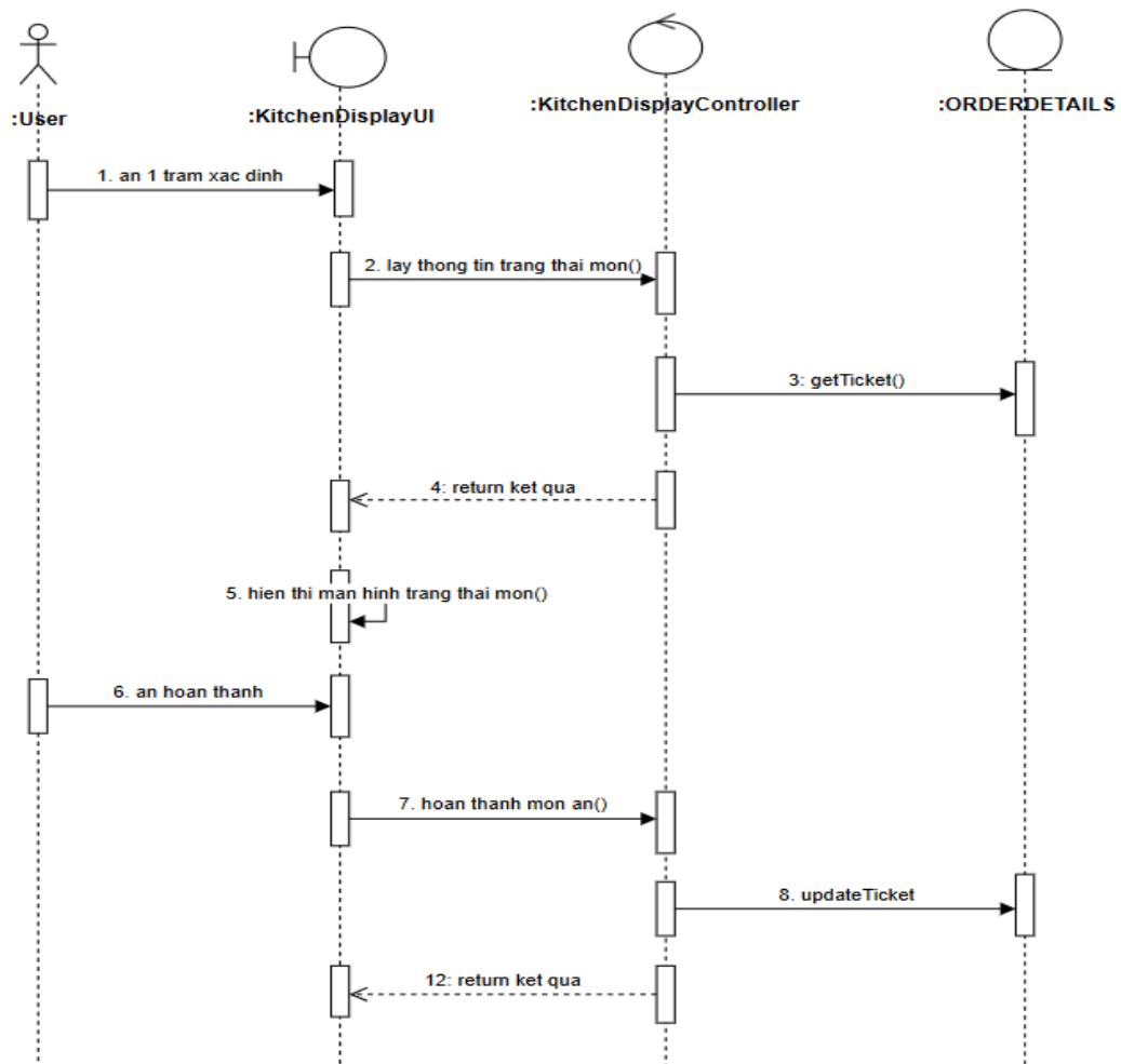
Hình 2.24: Biểu đồ trình tự use case Quản lý trạng thái món ăn
