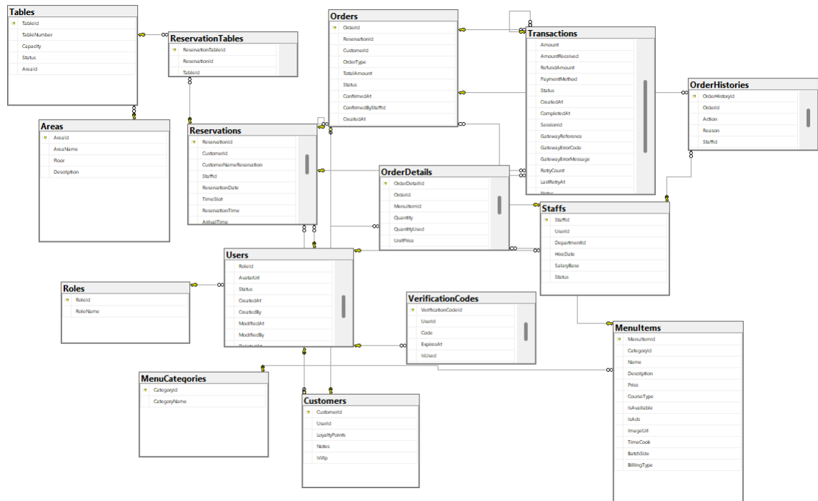
Hình 2.42: Cơ sở dữ liệu
