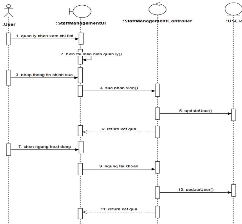
Hình 2.16: Biểu đồ trình tự use case Quản lý nhân viên
