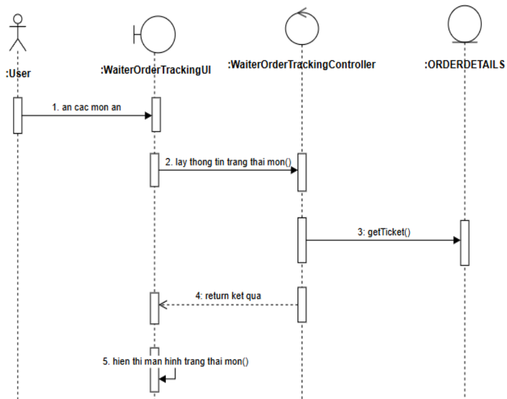
Hình 2.26: Biểu đồ trình tự use case Xem trạng thái món ăn
