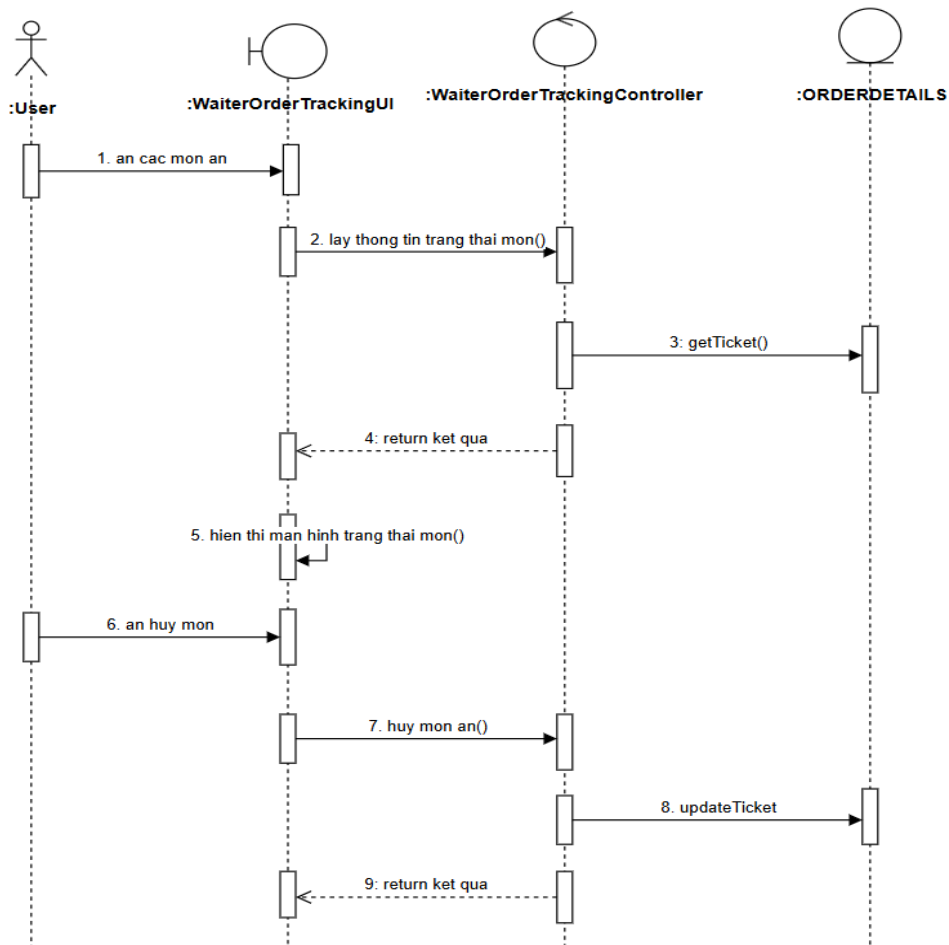
Hình 2.28: Biểu đồ trình tự use case Hủy món ăn
