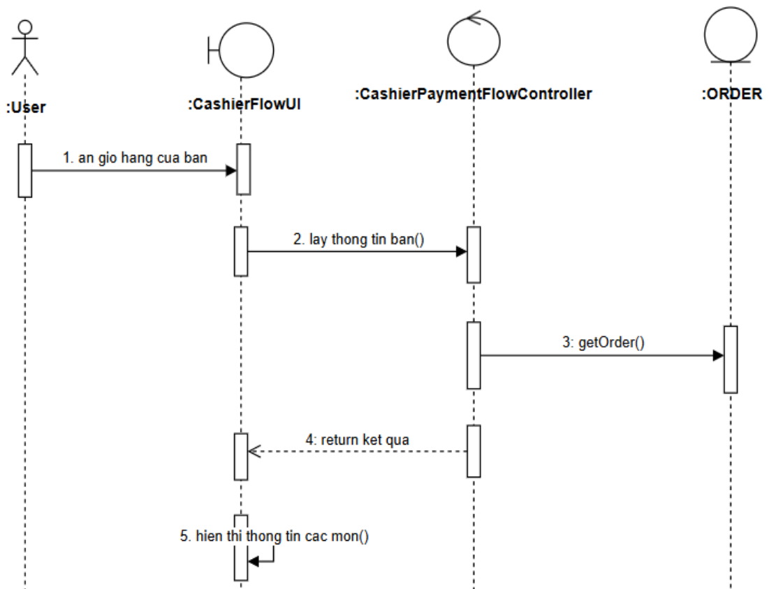
Hình 2.34: Biểu đồ trình tự use case Xem thông tin đặt món
