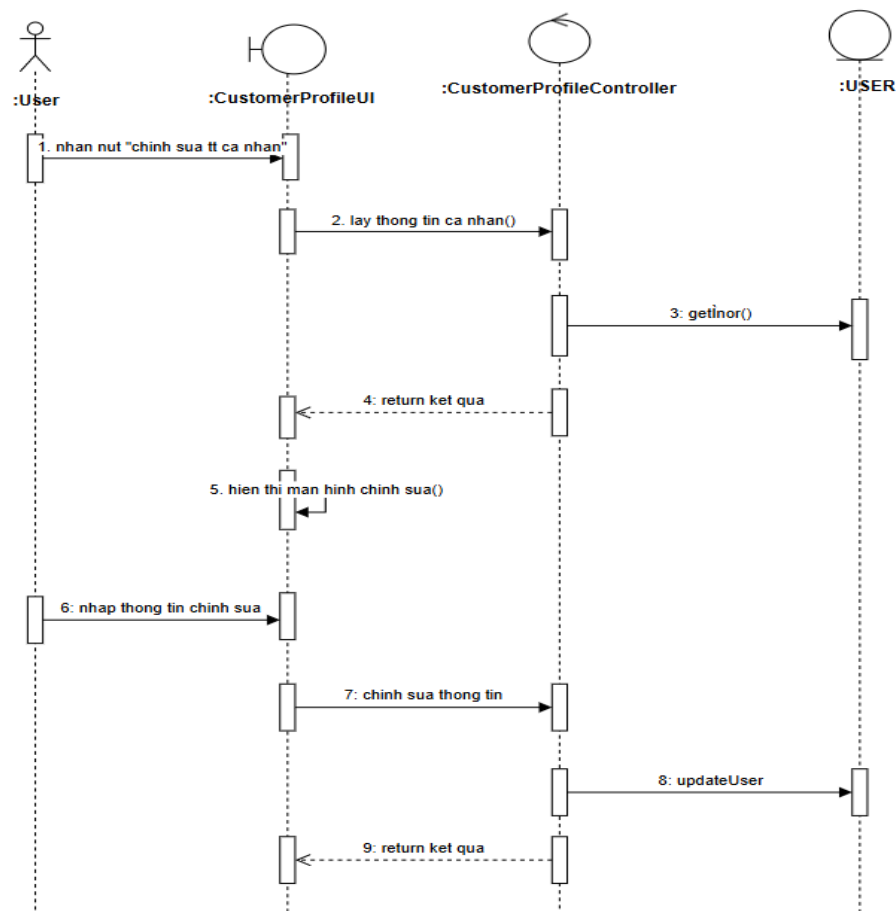
Hình 2.12: Biểu đồ trình tự use case Quản lý thông tin cá nhân
