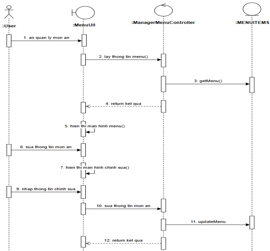
Hình 2.20: Biểu đồ trình tự use case Quản lý menu
