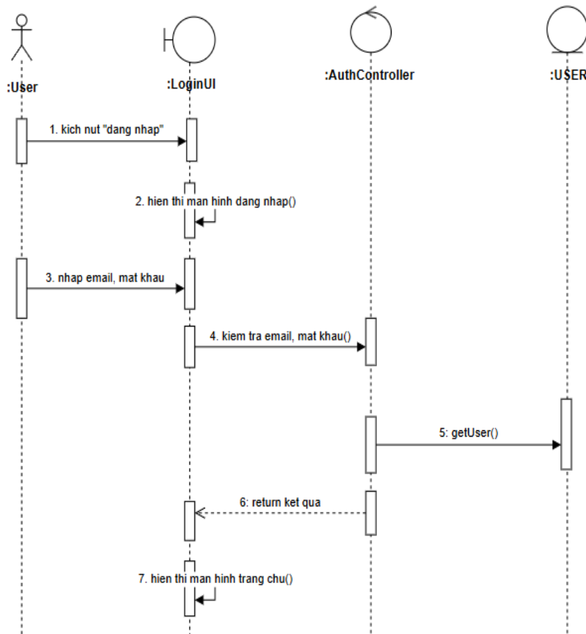
Hình 2.6: Biểu đồ trình tự use case Đăng nhập
