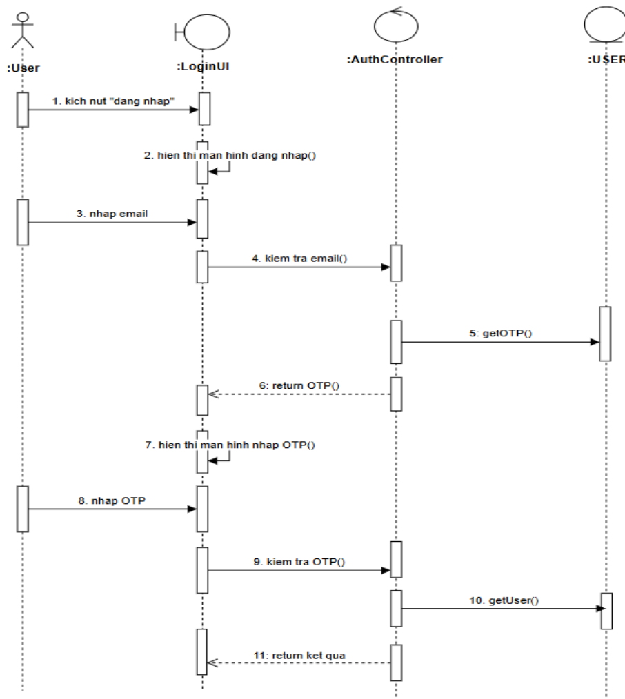
Hình 2.4: Biểu đồ trình tự use case Đăng nhập
