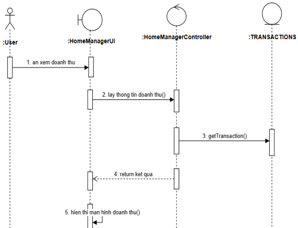
Hình 2.38: Biểu đồ trình tự use case Xem doanh thu
