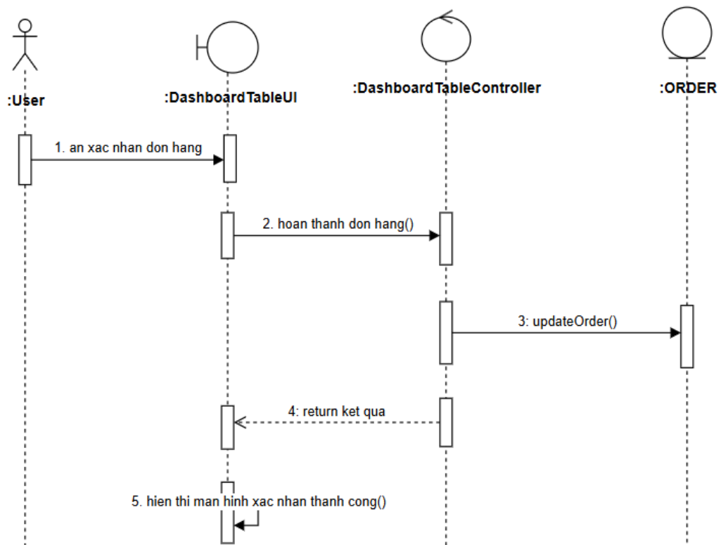
Hình 2.32: Biểu đồ trình tự use case Xác nhận đơn đặt món
