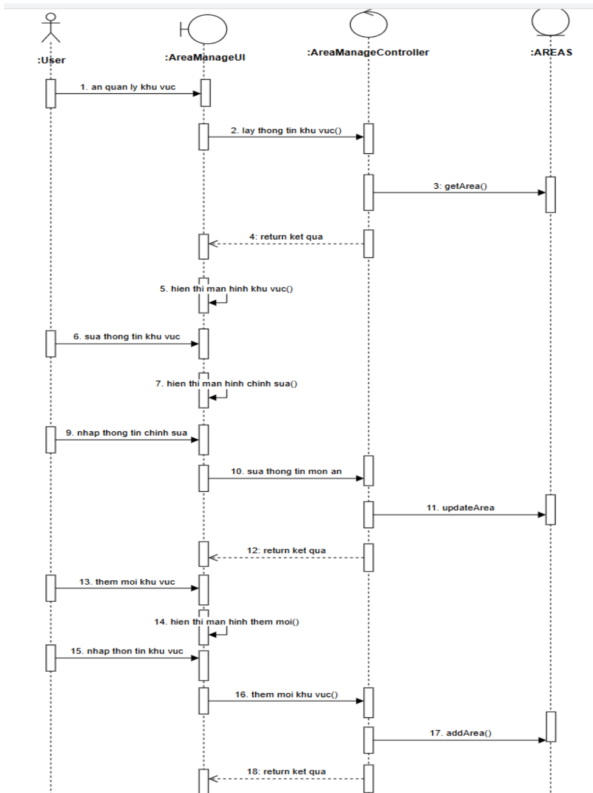
Hình 2.22: Biểu đồ trình tự use case Quản lý khu vực
