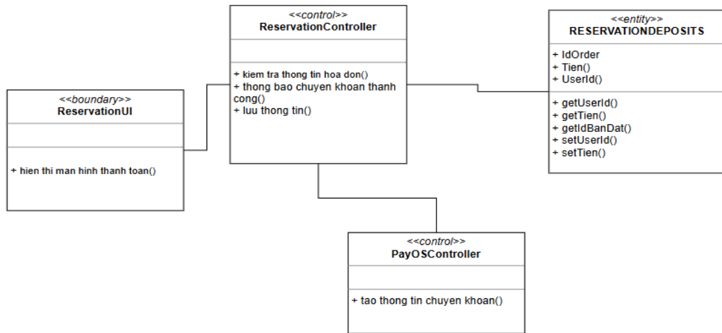
Hình 2.15: Biểu đồ VOPC use case Thanh toán
