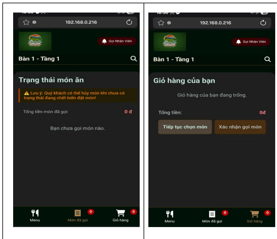
Hình 3.22: Giao diện quản lý các món ăn đã gọi của khách hàng
