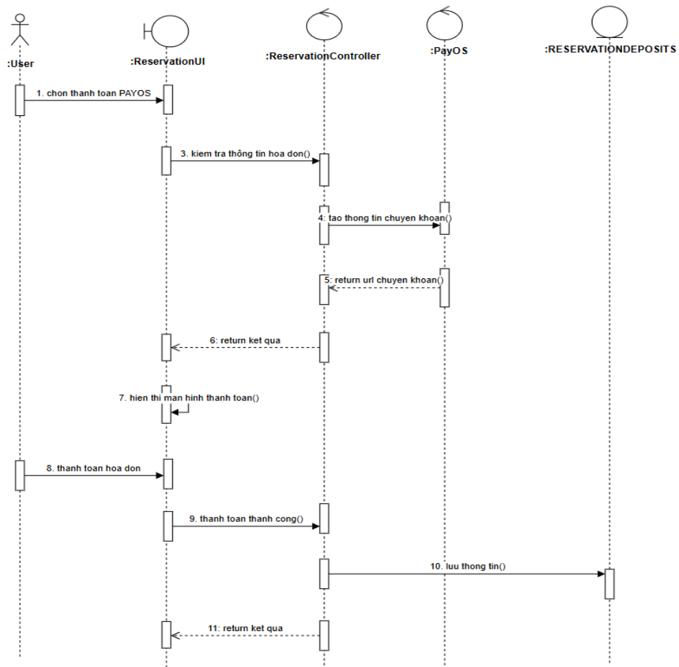
Hình 2.14: Biểu đồ trình tự use case Thanh toán
