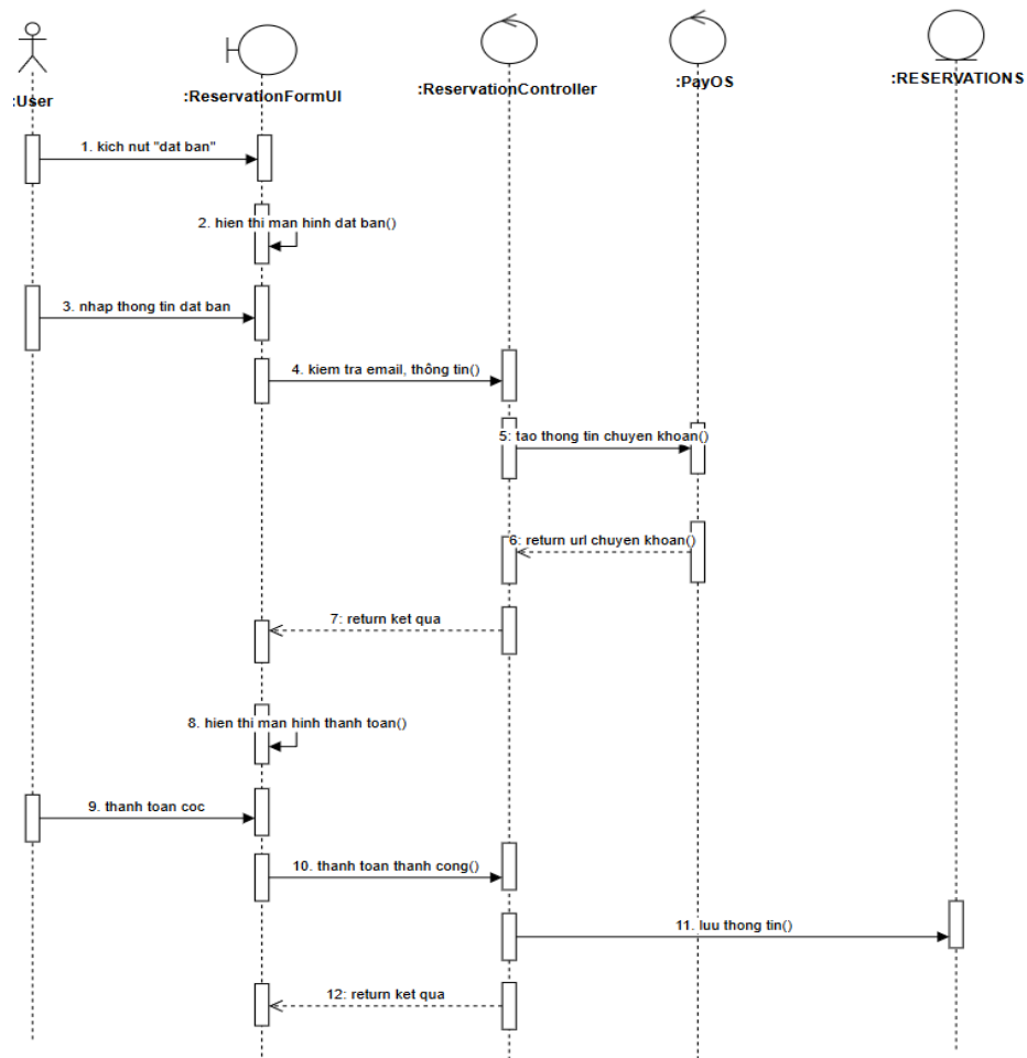
Hình 2.8: Biểu đồ trình tự use case Đặt bàn
