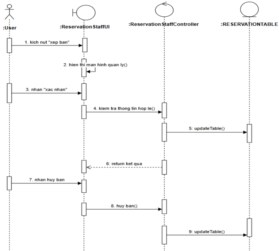
Hình 2.18: Biểu đồ trình tự use case Quản lý bàn đặt
