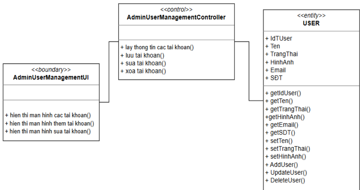
Hình 2.41: Biểu đồ VOPC use case Quản lý tài khoản
