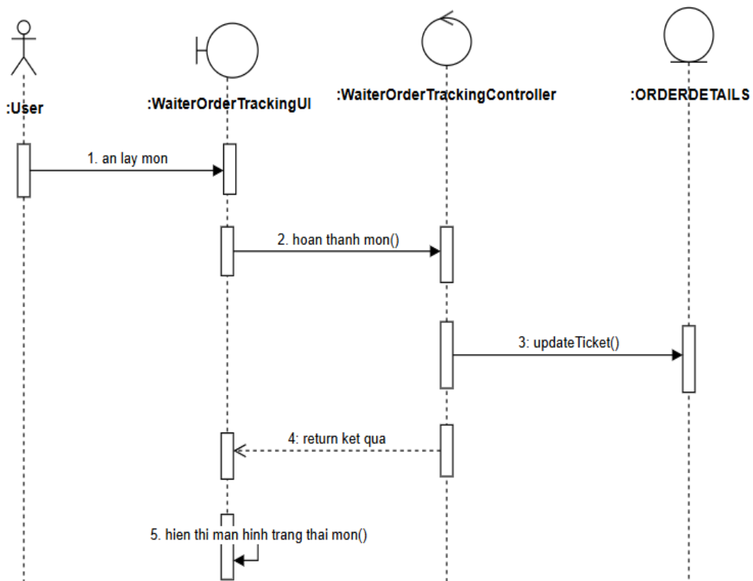
Hình 2.30: Biểu đồ trình tự use case Cập nhật trạng thái đơn đặt
