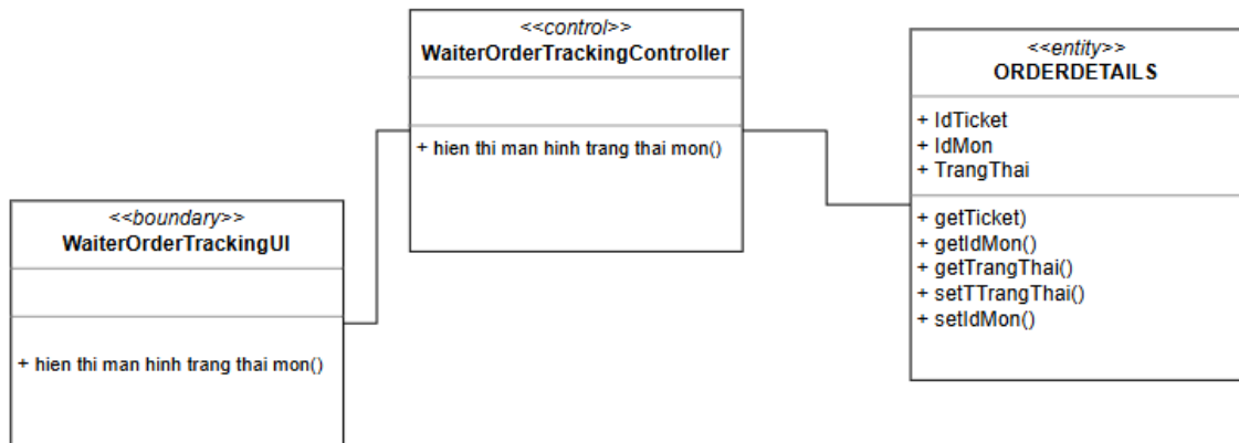
Hình 2.27: Biểu đồ VOPC use case Xem trạng thái món ăn
