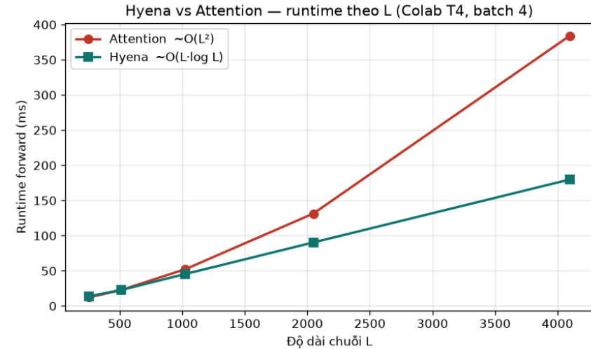
Runtime forward theo độ dài chuỗi L
