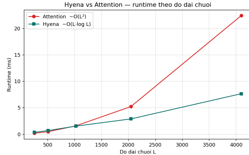
Runtime forward theo độ dài chuỗi L
