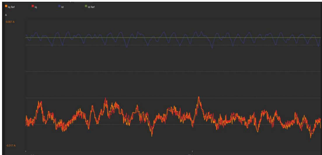
Hình 7.6: Đáp ứng bám dòng trục q trong khi duy trì dòng trục d xấp xỉ bằng không
