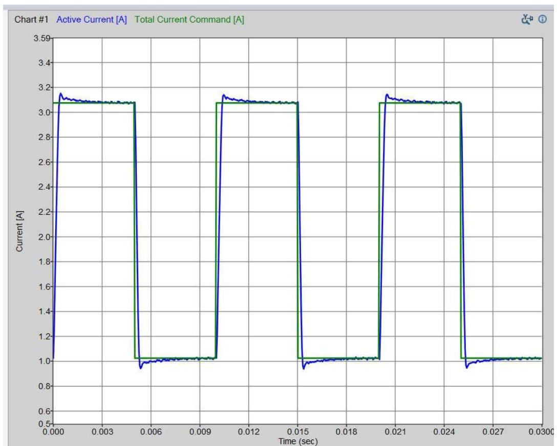
Hình 7.24: Đáp ứng bám dòng trực d với tín hiệu đặt xung vuông dùng driver thương mại khác
