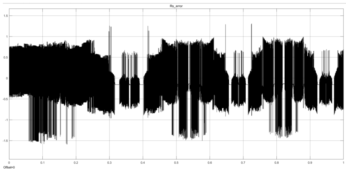
Hình 4.4: Kết quả mô phỏng ước lượng điện trở stator ( R_s ) – đồ thị sai số R\_estimate so với R_s \Omega .
