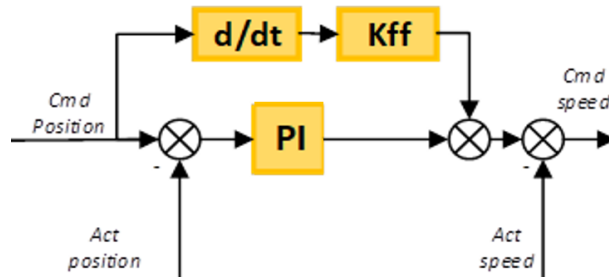
Hình 2.8: FeedForward trong sơ đồ điều khiển FOC
