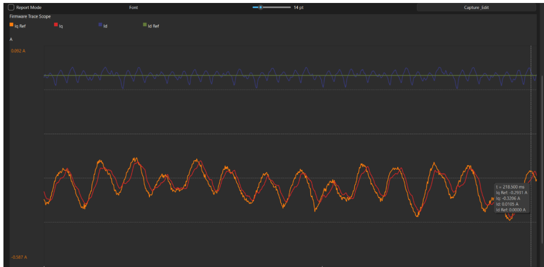
Hình 7.6: Đáp ứng bám dòng trục q trong khi duy trì dòng trục d xấp xỉ bằng không
