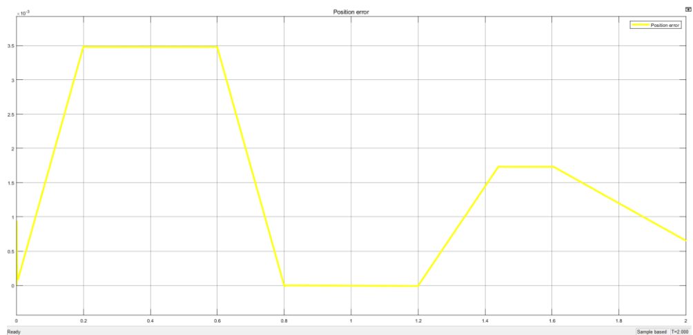
Hình 3.9: Sai số vị trí rotor ( \theta ) khi feed forward gain bằng 1 có tải
