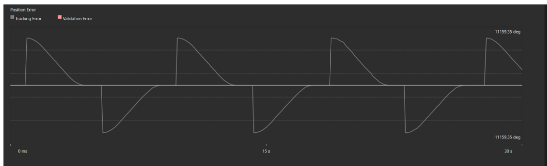
Hình 7.22: Đồ thị sai số bám vị trí trong bài kiểm tra qua lại hệ có tải.
