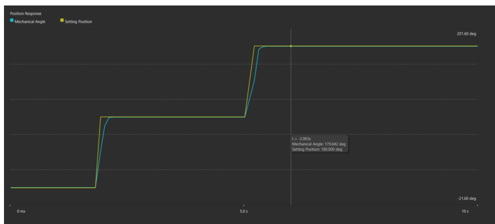
Hình 7.15: Đáp ứng vị trí của động cơ ở chế độ single-turn với tín hiệu đặt dạng bậc thang
