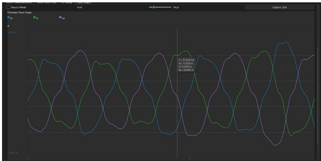
Hình 7.4: Dạng sóng dòng điện ba pha stator sau khi đóng vòng điều khiển dòng điện
