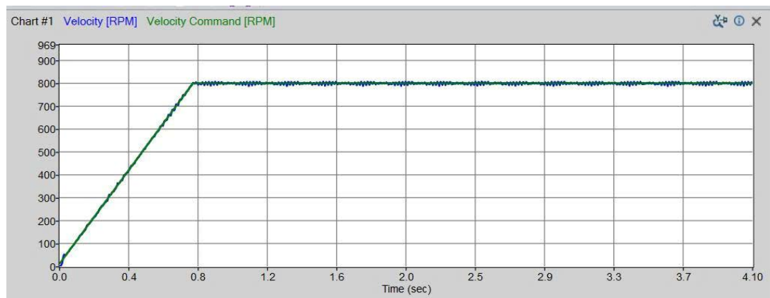
Hình 7.26: Đồ thị đáp ứng tốc độ có tải tại giá trị đặt 800 rpm
