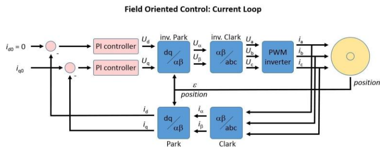
Hình 2.5: Sơ đồ khối vòng điều khiển dòng theo phương pháp FOC.
