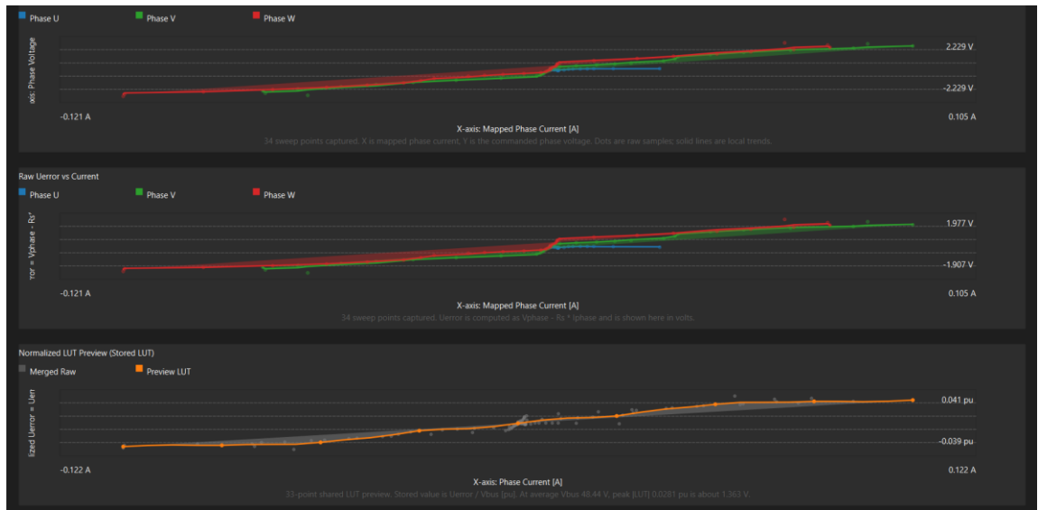
Hình 7.3: Kết quả đặc tính U_{error} theo dòng pha và LUT bù điện áp chuẩn hóa của động cơ
