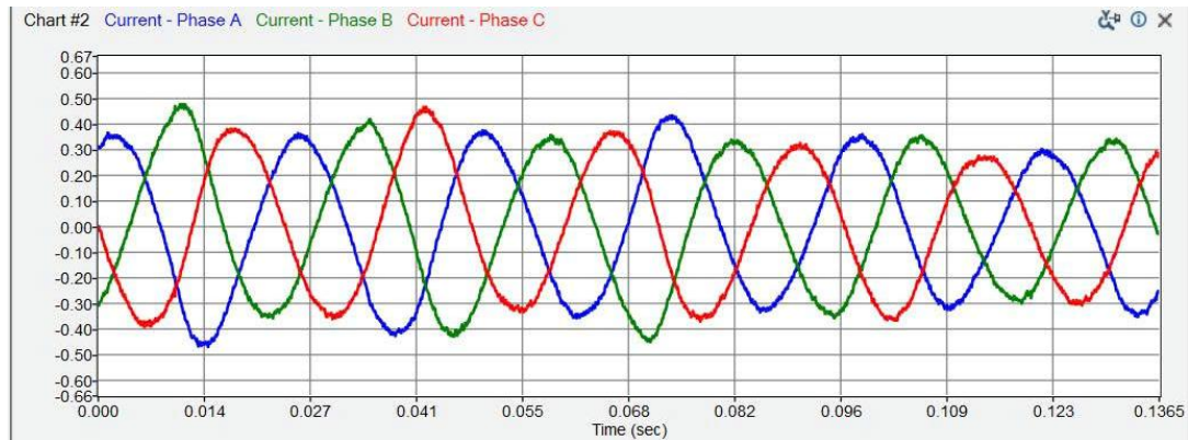
Hình 7.23: Dạng sóng dòng điện ba pha stator sau khi đóng vòng điều khiển dòng điện dùng driver thương mại khác
