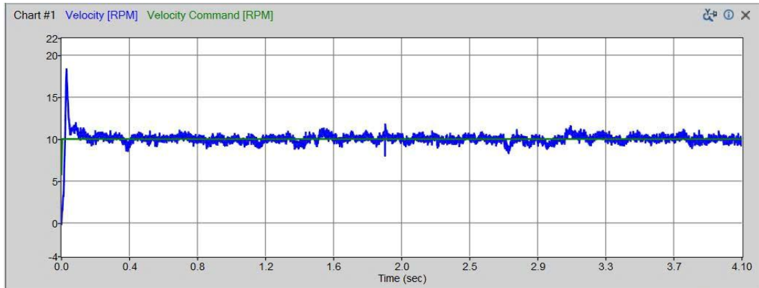
Hình 7.28: Đồ thị đáp ứng tốc độ có tải tại giá trị đặt 10 rpm dùng driver thương mại khác
