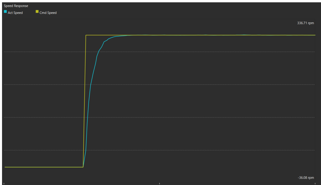
Hình 7.12: Đồ thị đáp ứng tốc độ không tải tại giá trị đặt 300 rpm
