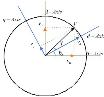
Hình 2.4: dq-transformation
