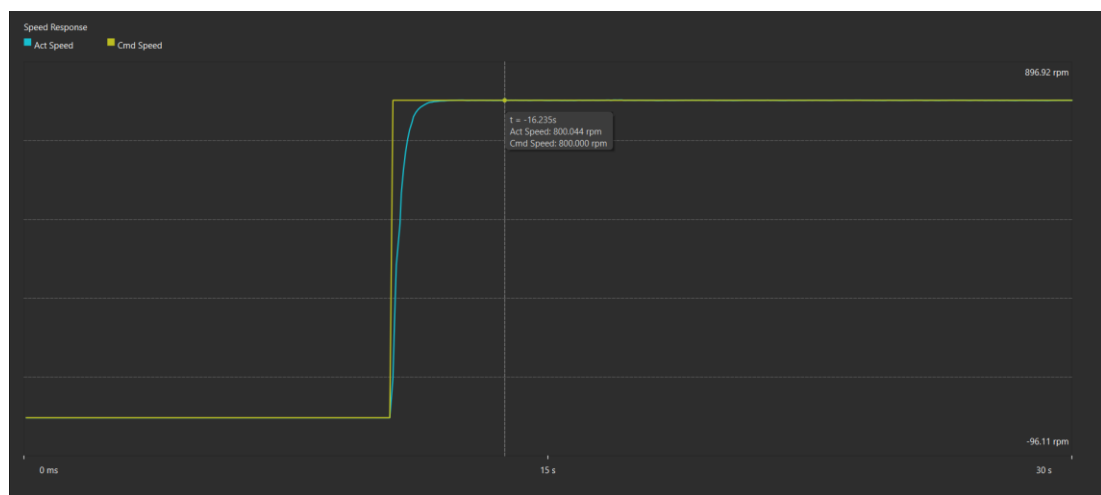
Hình 7.11: Đồ thị đáp ứng tốc độ không tải tại giá trị đặt 800 rpm
