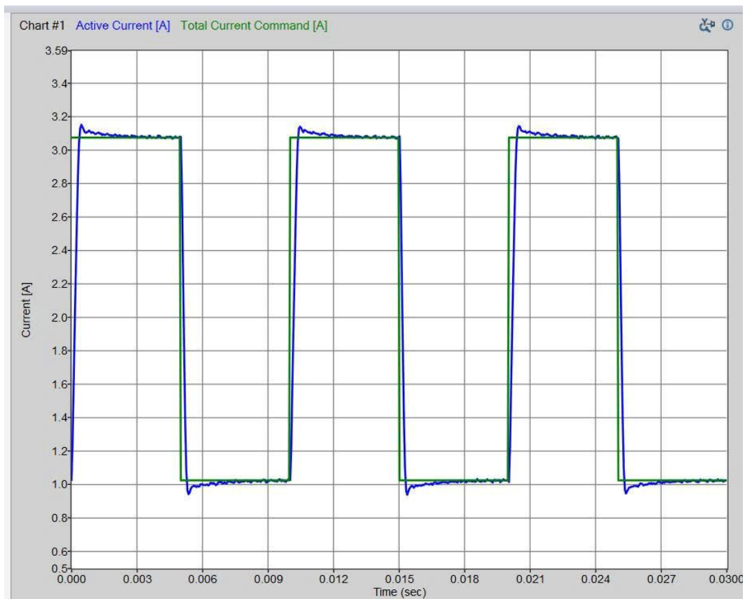
Hình 7.24: Đáp ứng bám dòng trục d với tín hiệu đặt xung vuông dùng driver thương mại khác
