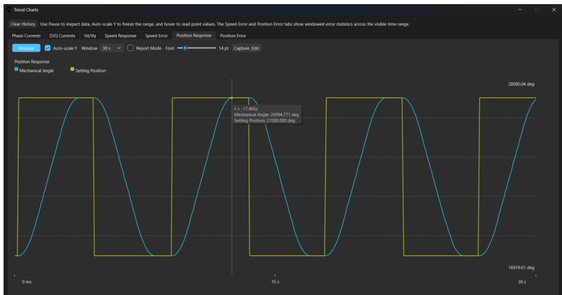
Hình 7.21: Đáp ứng vị trí qua lại giữa hai vị trí 180^\circ và 270^\circ trong 10 chu kỳ hệ có tải
