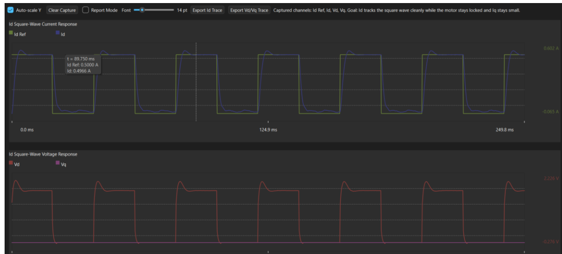
Hình 7.5: Đáp ứng bám dòng trục d với tín hiệu đặt xung vuông và điện áp điều khiển tương ứng
