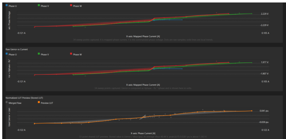
Hình 7.2: Kết quả đặc tính U_{error} theo dòng pha và LUT bù điện áp chuẩn hóa của động cơ ở chế độ không tải
