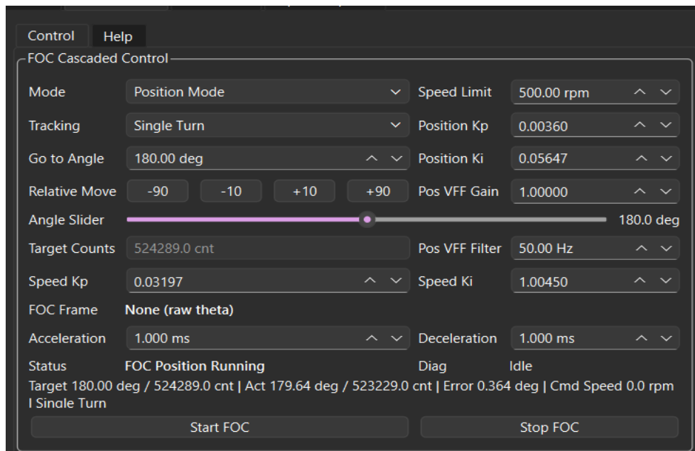
Hình 7.10: Giao diện cài đặt bộ điều khiển vị trí không tải của động cơ Panasonic ở chế độ single-turn
