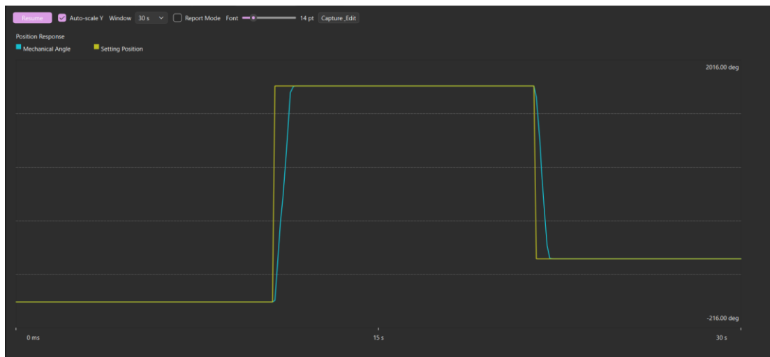
Hình 7.12: Đáp ứng vị trí của động cơ ở chế độ multi-turn
