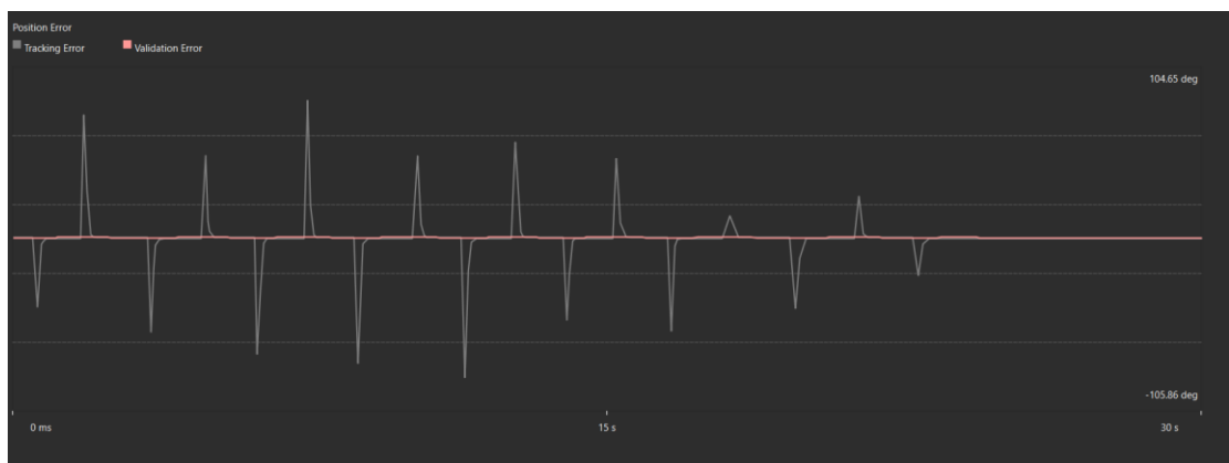
Hình 7.14: Đồ thị sai số bám vị trí trong bài kiểm tra qua lại.
