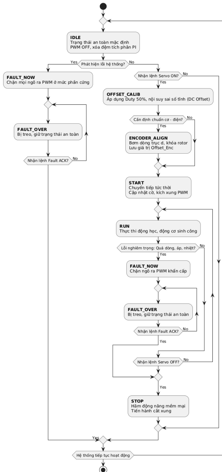
Hình 6.2: Sơ đồ luồng chuyển đổi trạng thái FSM của hệ thống Firmware
