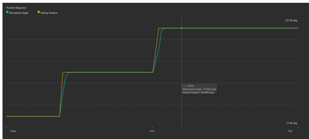
Hình 7.11: Đáp ứng vị trí của động cơ ở chế độ single-turn với tín hiệu đặt dạng bậc thang
