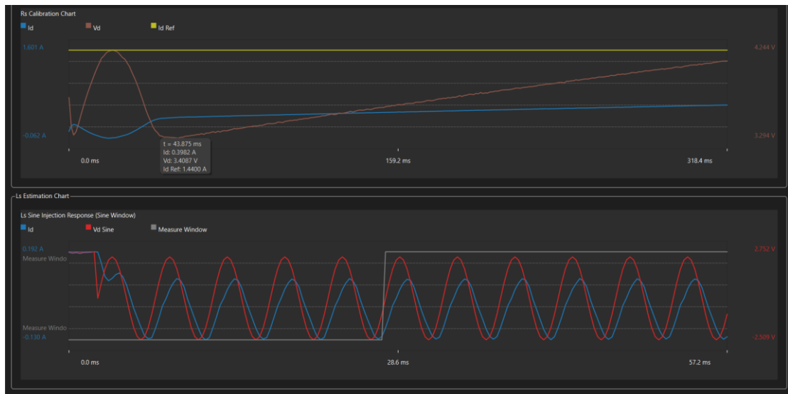
Hình 7.6: Đồ thị nhận dạng điện trở stator R_s (trên) và điện cảm stator L_s (dưới) trong quá trình Motor Auto-Tuning.
