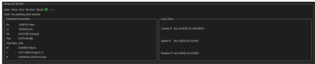
Hình 7.5: Kết quả ước lượng các tham số điện, cơ và hệ số PI sau khi hoàn tất quá trình Motor Auto-Tuning.
