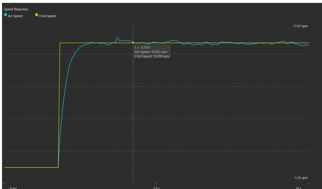
Hình 7.9: Đồ thị đáp ứng tốc độ không tải tại giá trị đặt 10 rpm
