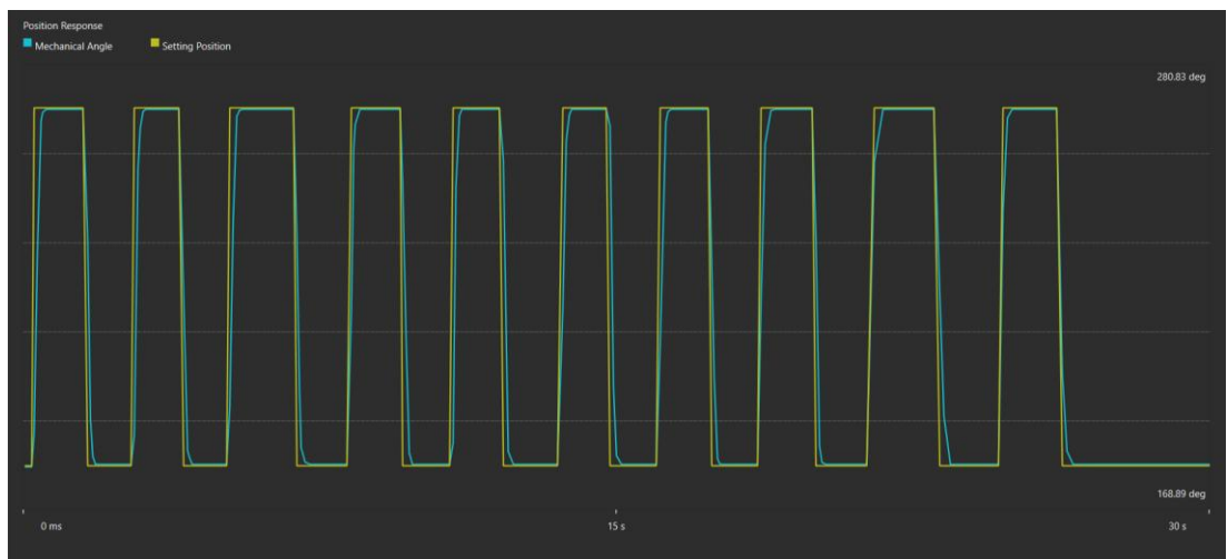
Hình 7.13: Đáp ứng vị trí qua lại giữa hai vị trí 180^\circ và 270^\circ trong 10 chu kỳ
