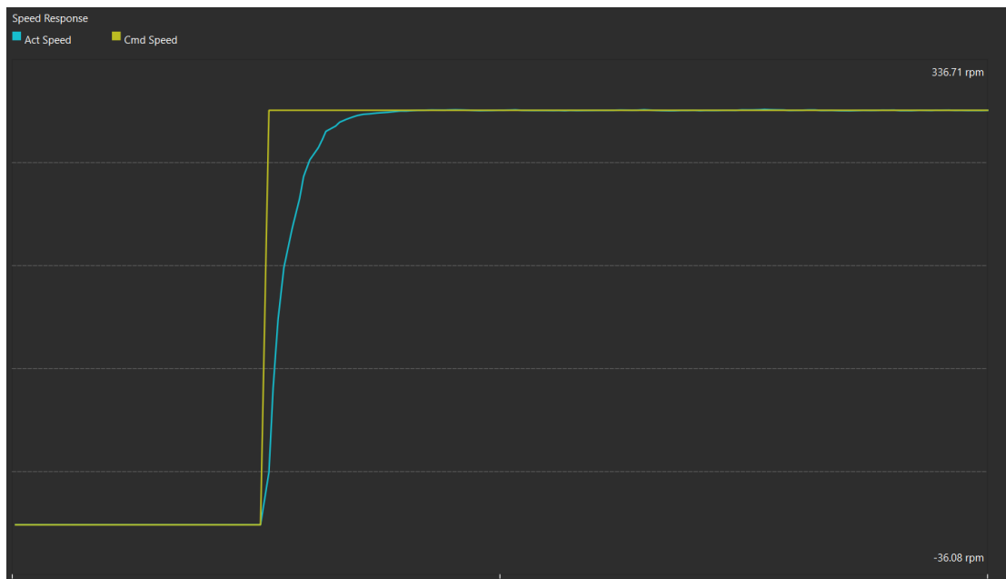
Hình 7.8: Đồ thị đáp ứng tốc độ không tải tại giá trị đặt 300 rpm
