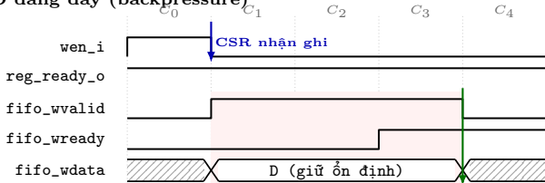
(b) FIFO đang đầy (backpressure)
