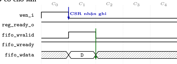
(a) FIFO có chỗ sẵn
