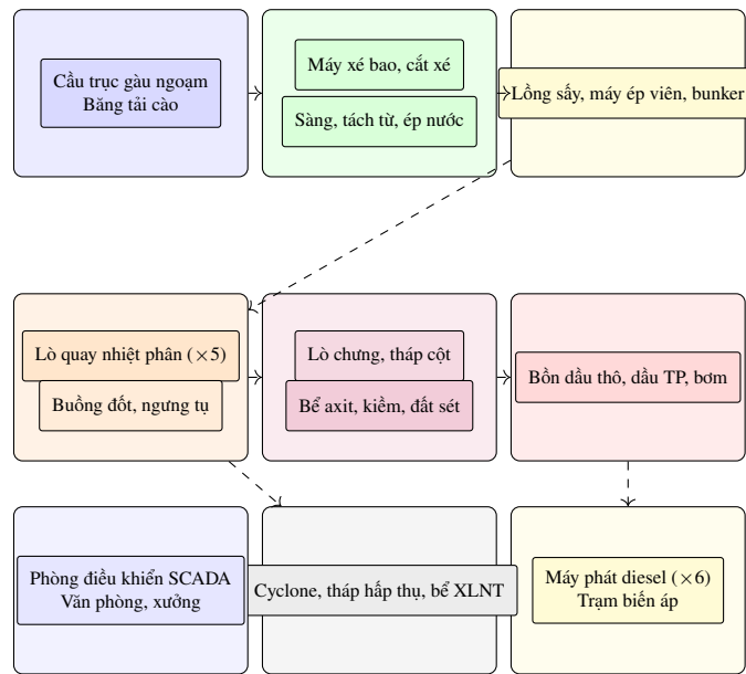
Hình 4.1: Sơ đồ bố trí mặt bằng công nghệ và các cụm thiết bị chính
