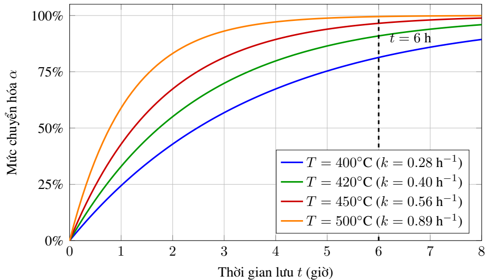
Hình 2.5: Đường cong chuyển hóa \alpha(t) = 1 - \exp(-k \cdot t) tại các nhiệt độ vận hành khác nhau
