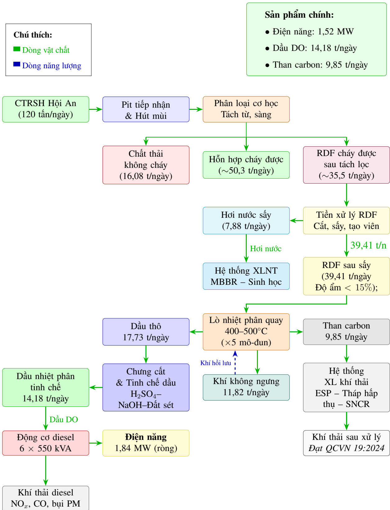
Hình 3.1: Sơ đồ dòng chảy công nghệ (PFD) tổng thể nhà máy nhiệt phân – chưng cất – phát điện diesel Hội An
