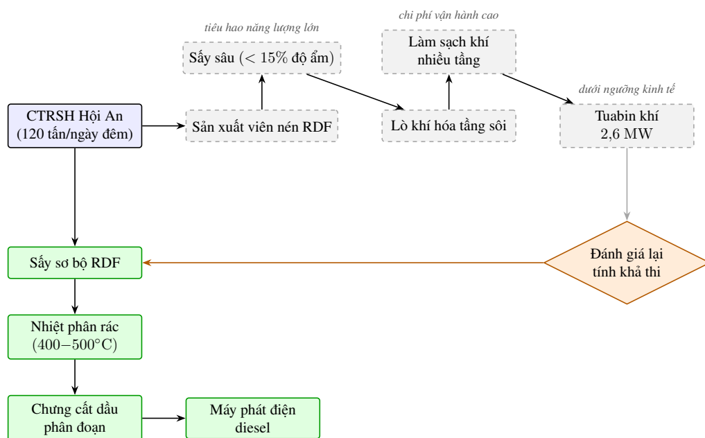
Hình 2.4: Chuyển đổi công nghệ xử lý CTRSH Hội An từ công nghệ khí hóa sang công nghệ nhiệt phân
