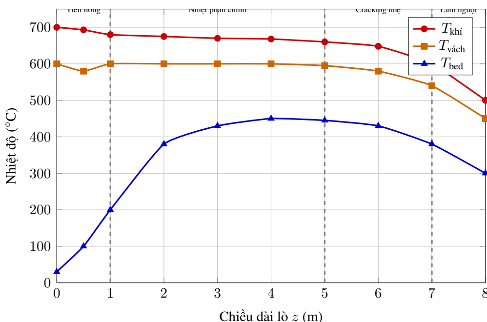
Hình 3.7: Biên dạng phân bố nhiệt độ dọc theo chiều dài lò nhiệt phân quay ( L = 8 m)
