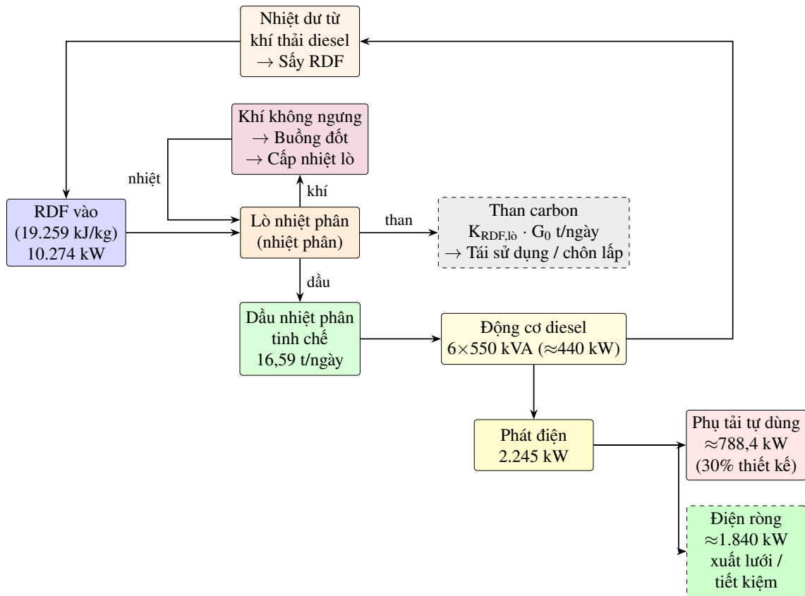
Hình 3.5: Sơ đồ tích hợp dòng năng lượng trong nhà máy
