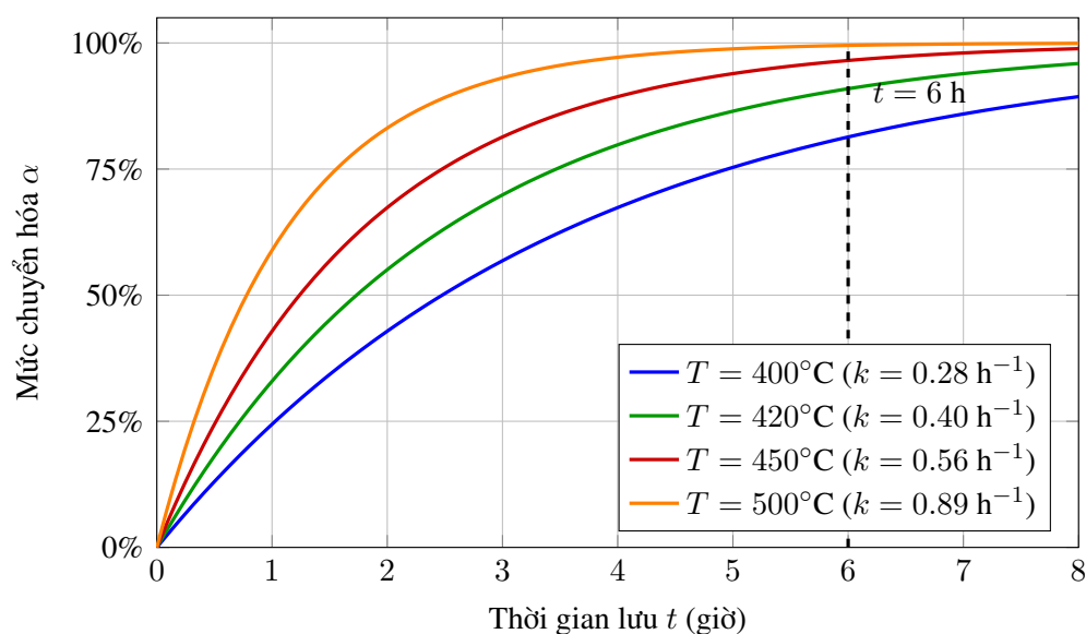
Hình 2.3: Đường cong chuyển hóa \alpha(t) = 1 - \exp(-k \cdot t) tại các nhiệt độ vận hành khác nhau
