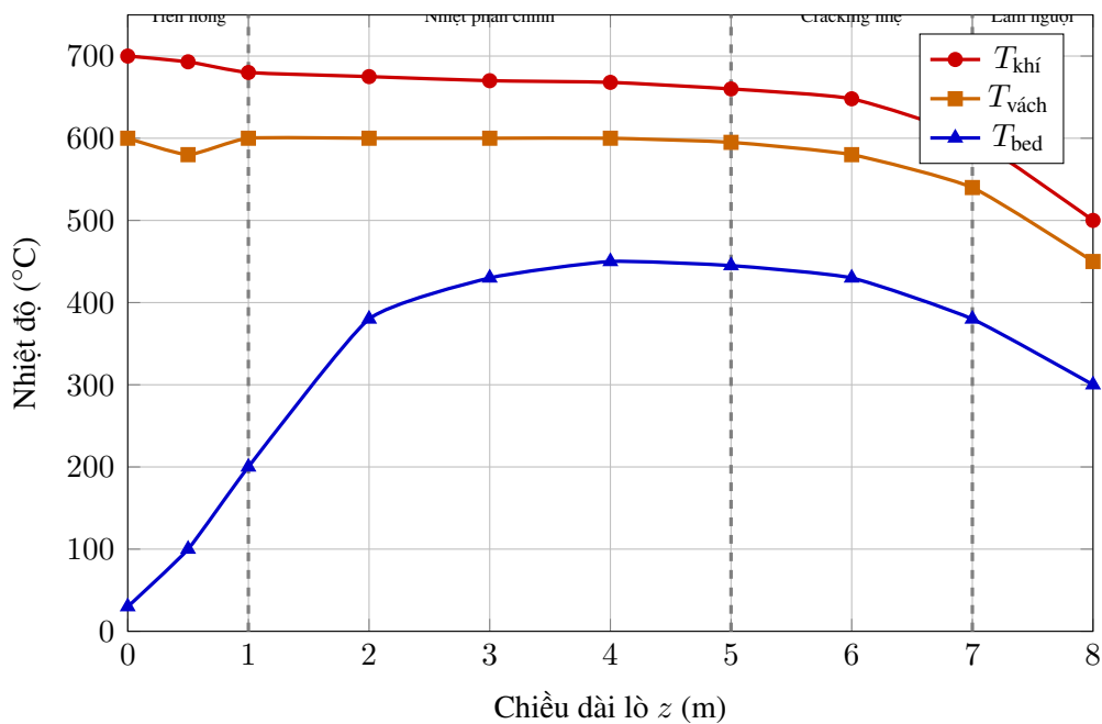
Hình 4.2: Biên dạng phân bố nhiệt độ dọc theo chiều dài lò nhiệt phân quay ( L = 8 m)
