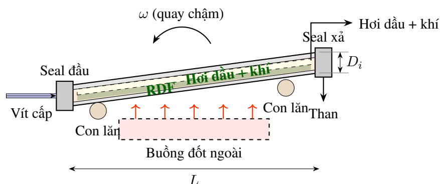
Hình 2.3: Nguyên lý lò nhiệt phân quay
