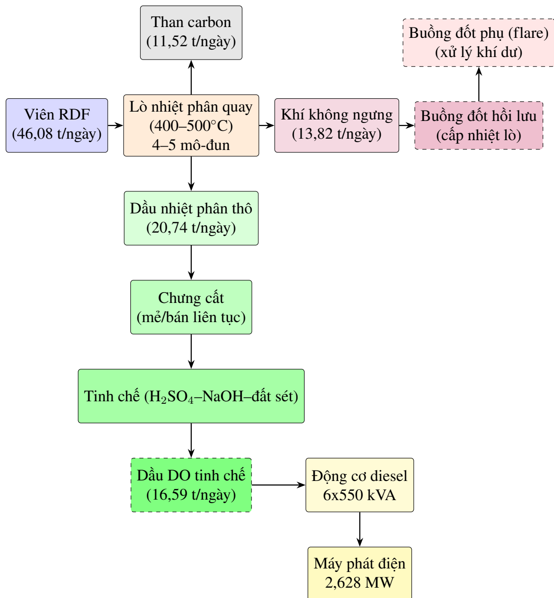
Hình 2.5: Sơ đồ công nghệ tổng thể của phương án nhiệt phân – chưng cất – phát điện diesel
