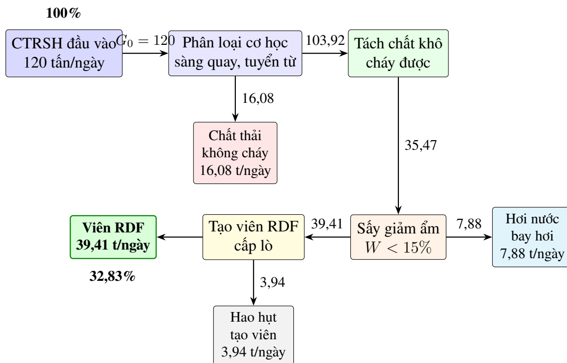
Hình 3.2: Sơ đồ cân bằng vật chất khối tiền xử lý và sản xuất RDF
