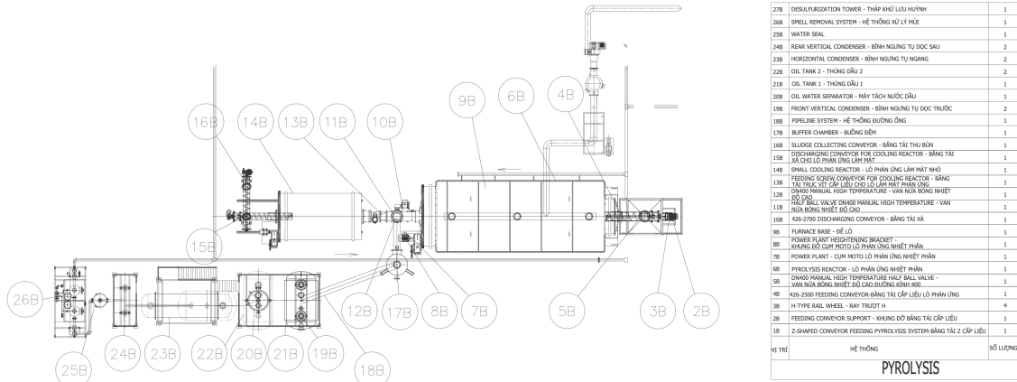
Hình 3.8: Bản vẽ hệ thống nhiệt phân và danh mục thiết bị
