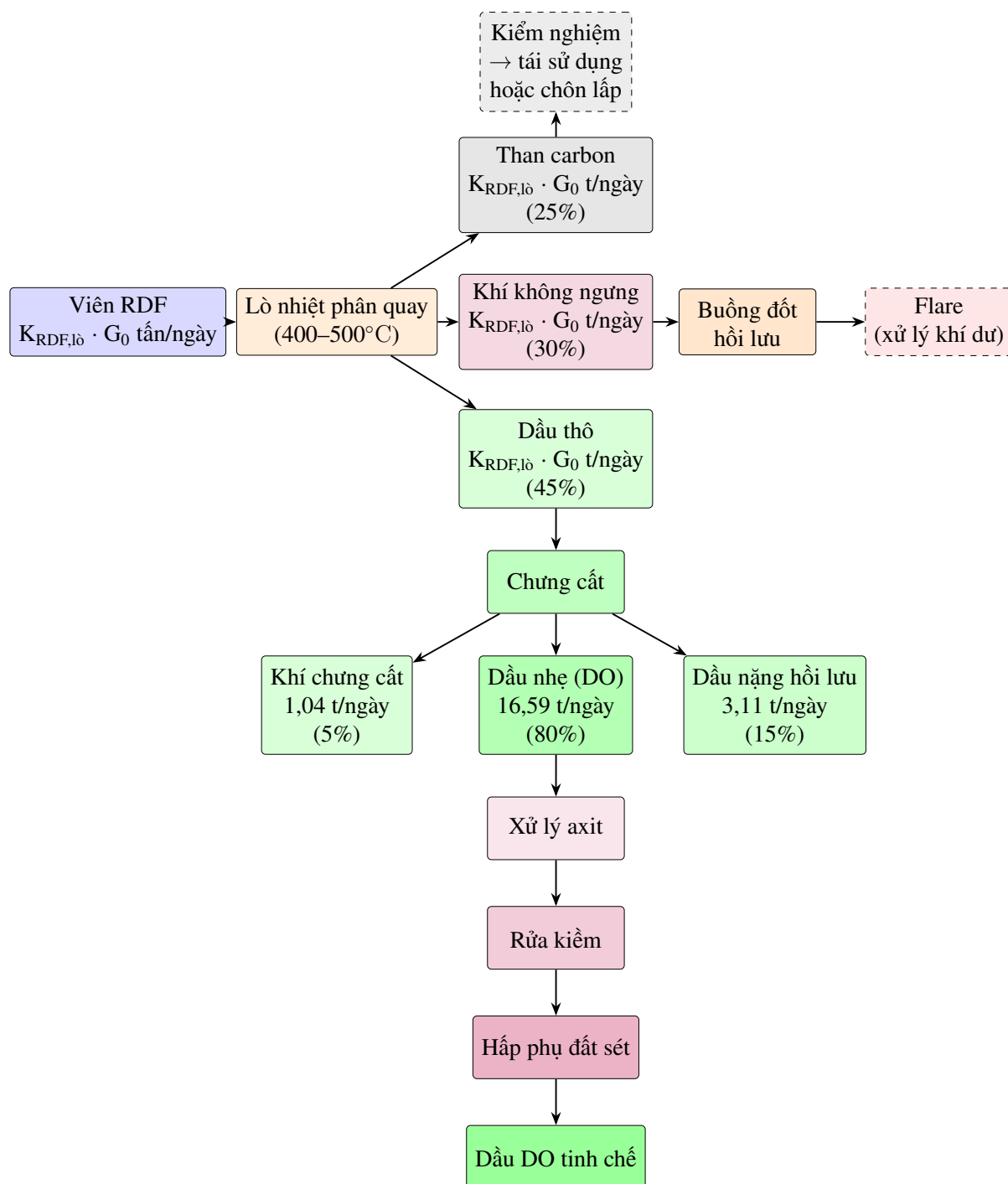
Hình 3.3: Sơ đồ cân bằng dòng sản phẩm của khối nhiệt phân và chưng cất
