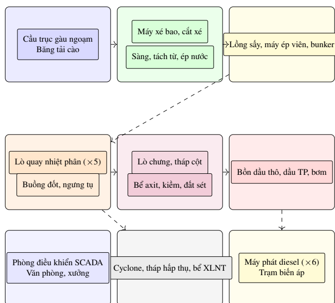
Hình 3.6: Sơ đồ bố trí mặt bằng công nghệ và các cụm thiết bị chính
