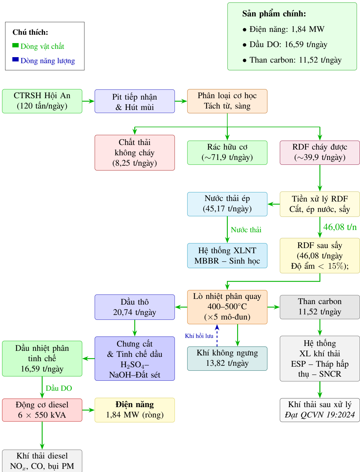
Hình 3.5: Sơ đồ dòng chảy công nghệ (PFD) tổng thể nhà máy nhiệt phân – chưng cất – phát điện diesel Hội An
