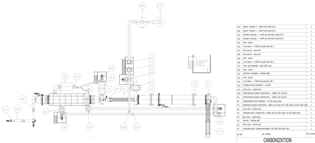
Hình 3.8: Bản vẽ hệ thống than carbon và danh mục thiết bị
