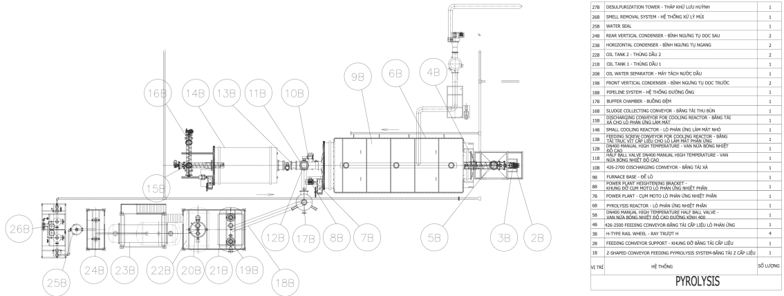
Hình 3.7: Bản vẽ hệ thống nhiệt phân và danh mục thiết bị
