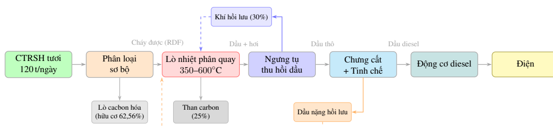
Hình 2.5: Sơ đồ công nghệ tổng thể: tiền xử lý – nhiệt phân – tinh chế – phát điện
