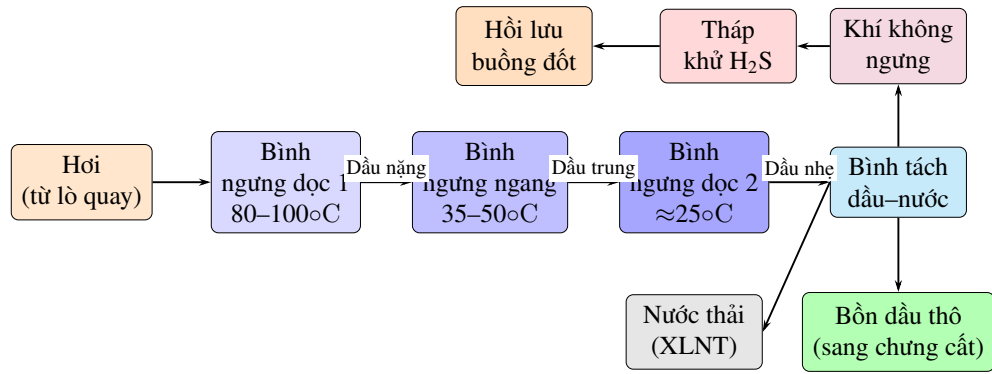
Hình 2.5: Sơ đồ hệ thống ngưng tụ thu hồi dầu ba cấp
