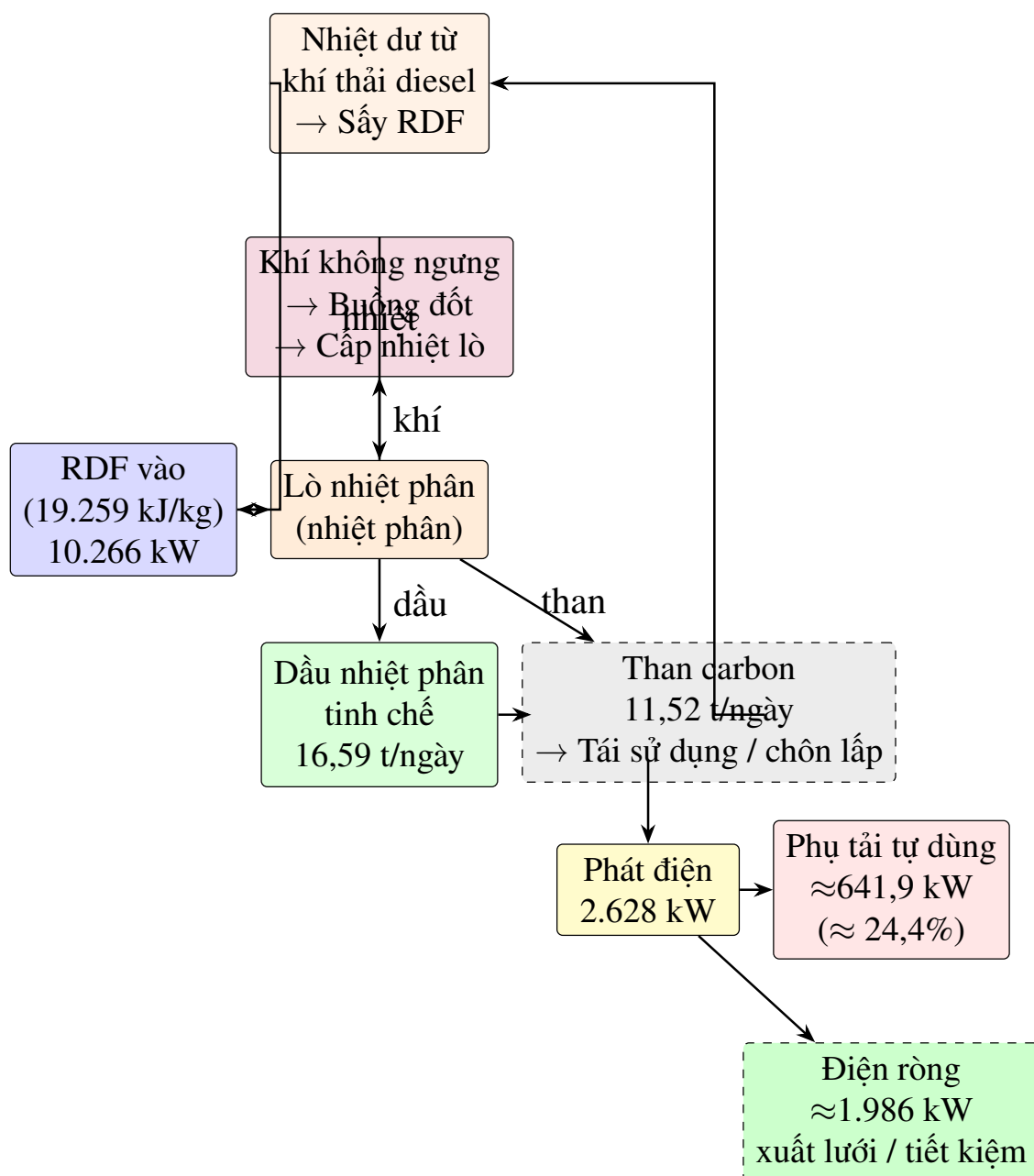
Hình 3.3: Sơ đồ tích hợp dòng năng lượng trong nhà máy
