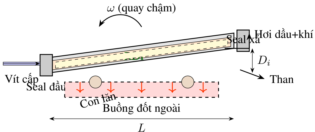
Hình 2.3: Nguyên lý lò nhiệt phân quay
