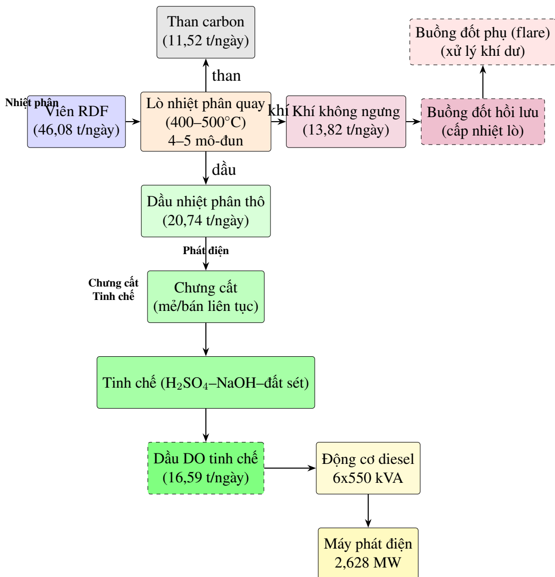
Hình 2.5: Sơ đồ công nghệ tổng thể của phương án nhiệt phân – chưng cất – phát điện diesel
