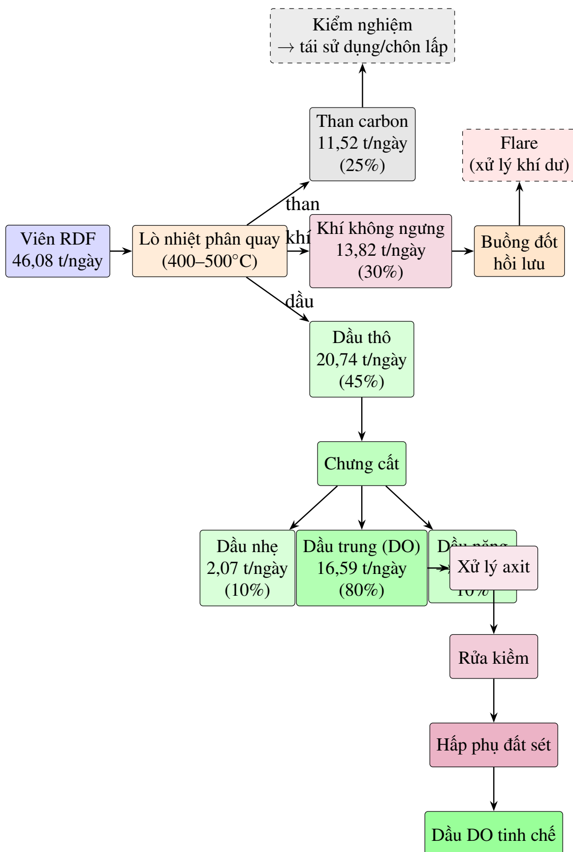
Hình 3.2: Sơ đồ cân bằng dòng sản phẩm của khối nhiệt phân và chưng cất
