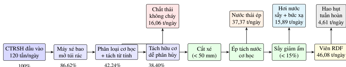
Hình 3.1: Sơ đồ cân bằng vật chất tổng thể khối tiền xử lý và sản xuất RDF
