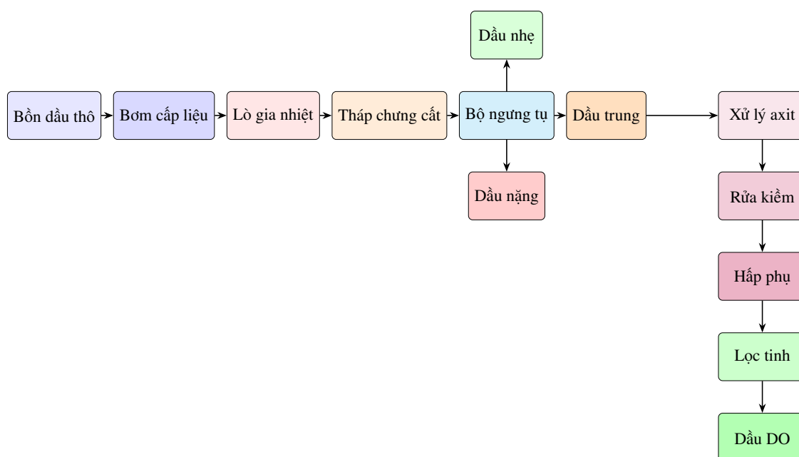
Hình 2.4: Sơ đồ chưng cất và tinh chế dầu
