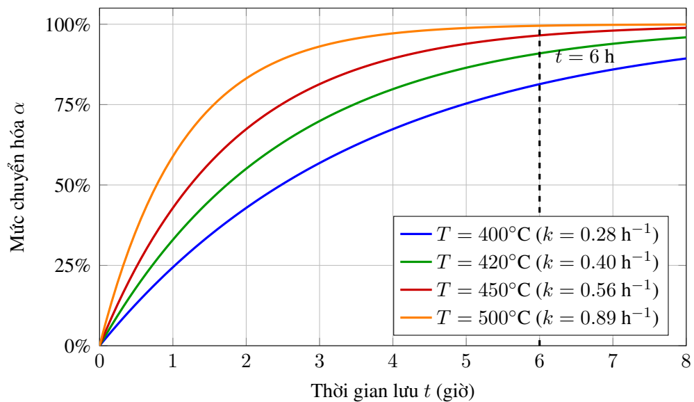
Hình 2.1: Đường cong chuyển hóa \alpha(t) = 1 - \exp(-k \cdot t) tại các nhiệt độ vận hành khác nhau
